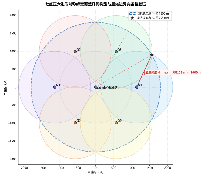
图 5 七点蜂窝全域完备覆盖几何验证
