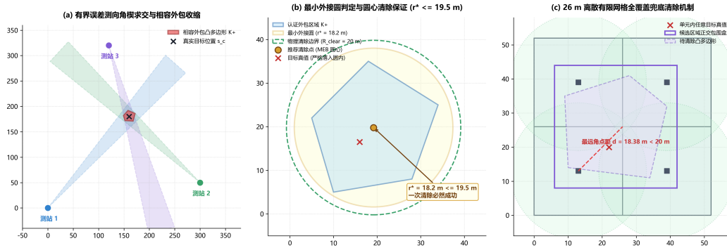
图 6 角楔交会、MEB 判据与网格兜底机制示意图
