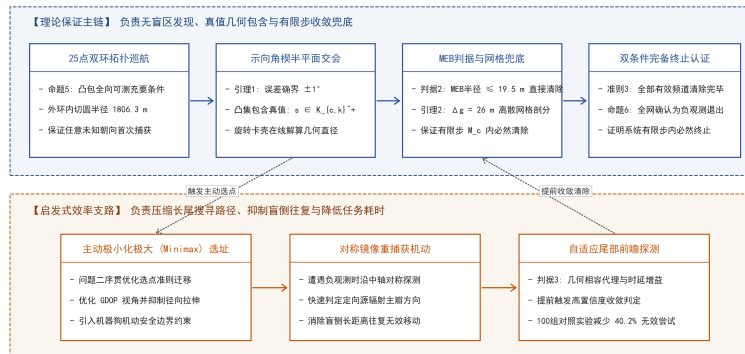
图 8 全向一定向混合干扰源自主协同搜索与清除系统架构图
