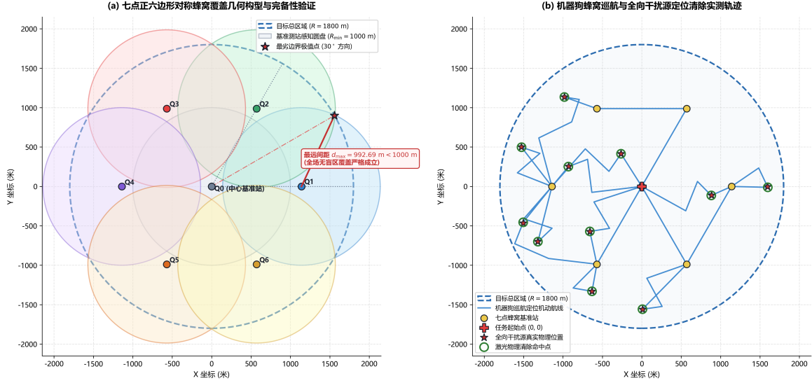
图 6 七点正六边形对称蜂窝全域覆盖几何构型 (a) 与机器狗巡航清除实测轨迹 (b)
