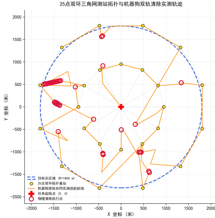
图 8 25 点双环拓扑分布构型与机器狗双轨清除实测轨迹
