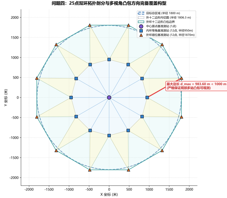
图 7 25 点双环测站拓扑分布与三角形覆盖构型
