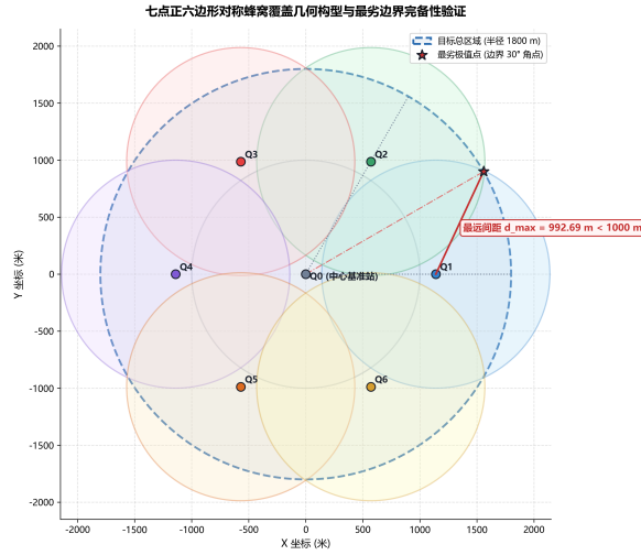
图 5 七点蜂窝全域完备覆盖几何验证
