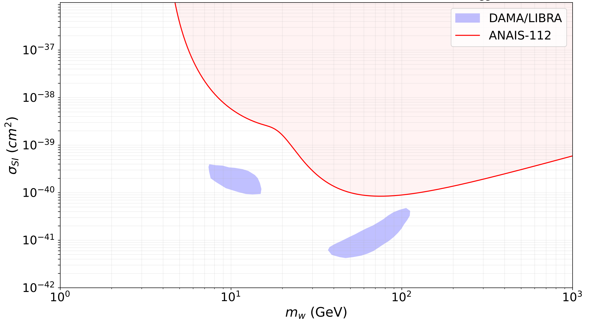
Curva de Exclusión - SI - Intervalo de 1 – 6 keV_{ee}
