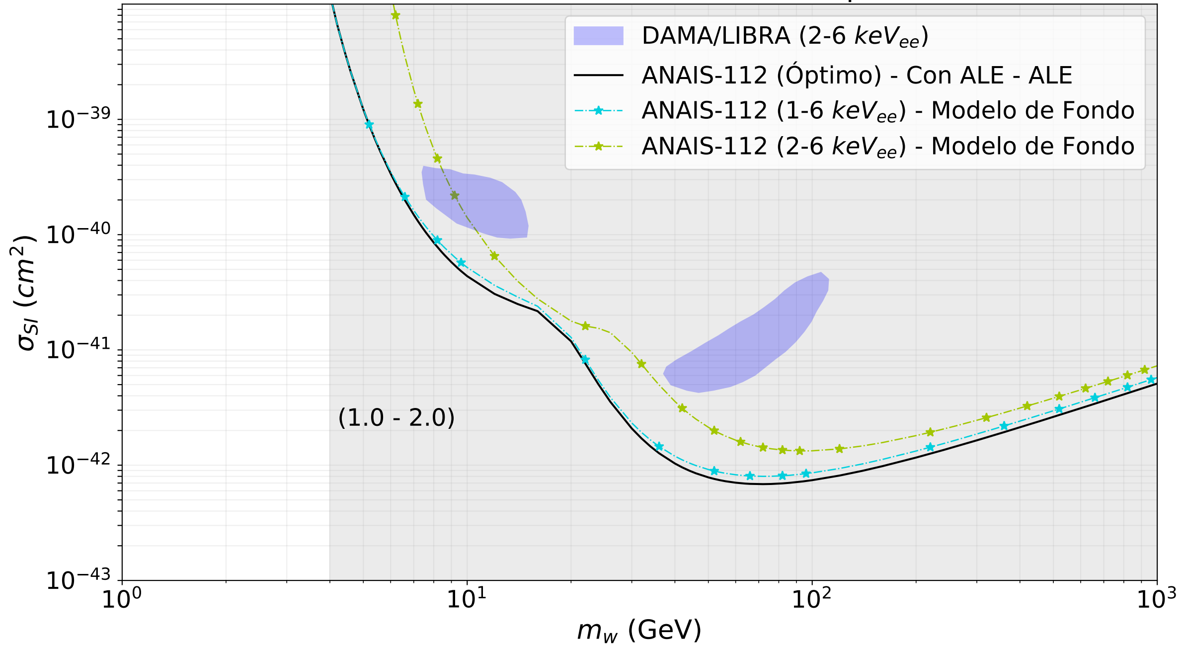
Plots de Exclusión - SI - Intervalo óptimo
