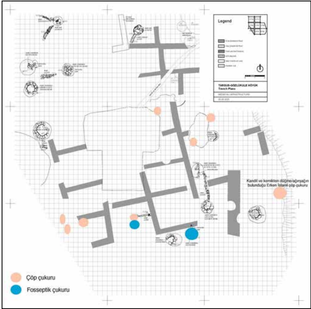
Plan 1: Tarsus-Gözlükule Höyük Orta Çağ katmanı Erken İslami Dönem yapı kalıntıları ve su gideri ile bağlanan alt yapıların şematik planı. Mimari plan: Figen Öztürk.
