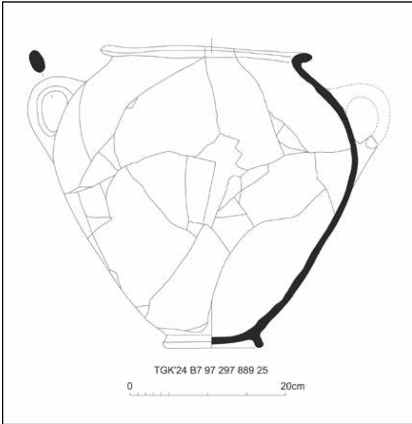
Çizim 4: B797 locus 297’de bulunan çift kulplu saklama kabı.
