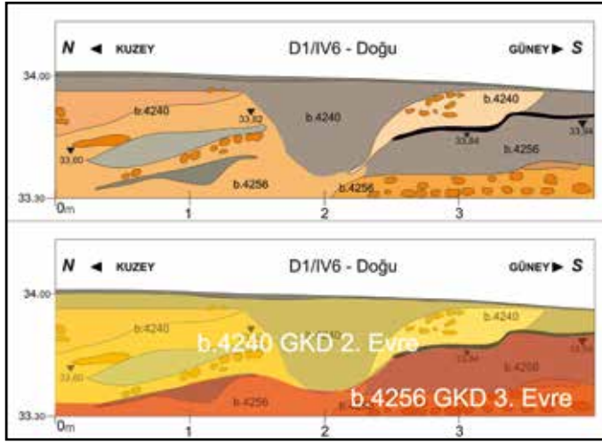
Çizim 3: Geç Kalkolitik Dönem 2. ve 3. Mimari Tabakaların kesit çizimleri.
