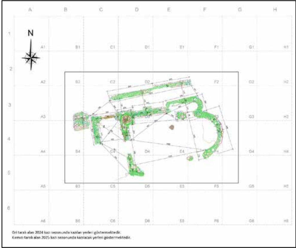
Çizim 1: Yuşa Tepesi Bizans Kilisesi'nin rölöve planı (Arkeo Teknik).
