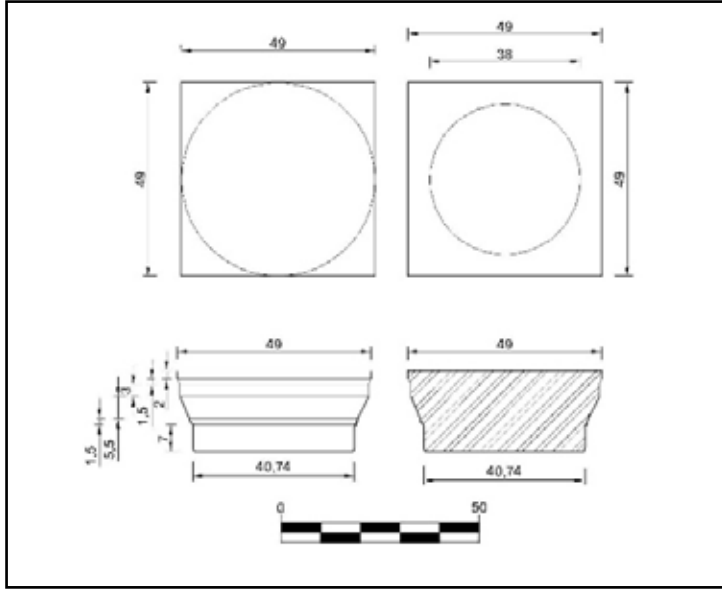
Resim 15a: Mimari belgeleme/çizim çalışmaları.
