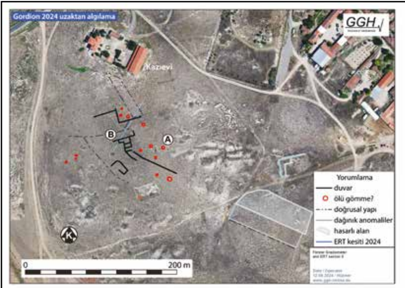
Resim 9: Kazı evinin güneyinde uzaktan algılama ile ortaya çıkarılan duvarların yorumlandığı planı. A: pithos gömüleri (?); B: çevre duvarı/giriş kapısı. Plan: GGH.
