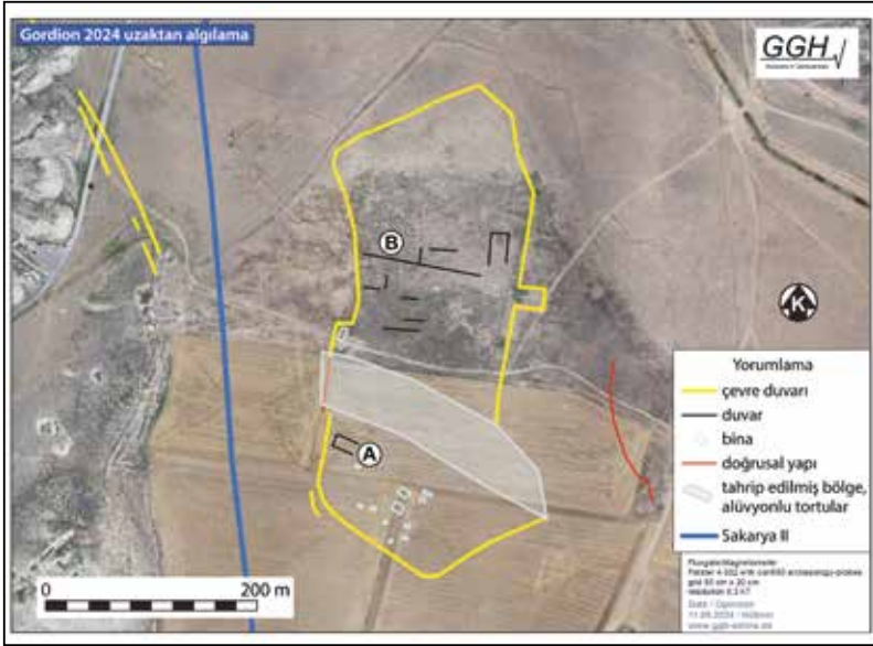
Resim 8: Doğu Dış Şehir ve çevresindeki surların 2024 yılında uzaktan algılamaya dayalı yorumsal planı. A: megaron ; B: avlu duvarları? Plan: GGH.
