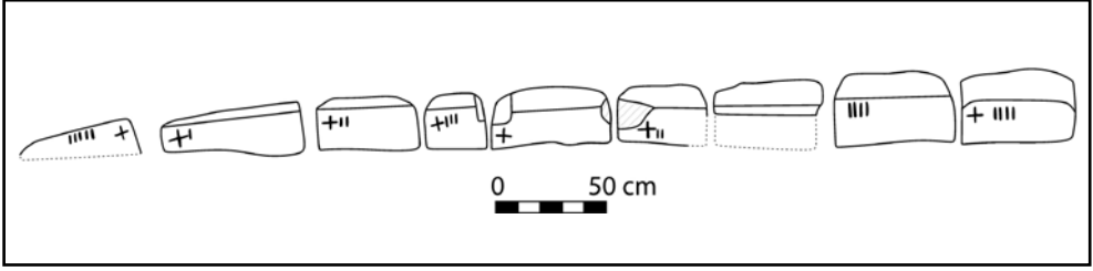
Resim 6: Mozaikli Bina Kompleksi'nin yeni keşfedilen güneybatı duvarındaki numaralandırma sistemi. Çizim: Ali Can Kırcaali.
