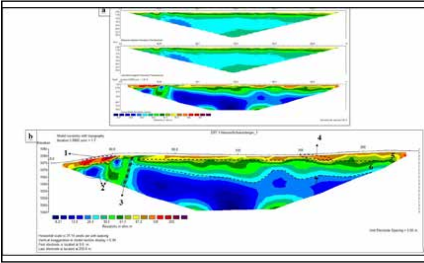
Resim 3: (a) Resim 2’de gösterilen 240 metre uzunluktaki birinci ERT profile ait ölçüm haritaları, (b) topoğrafik düzeltilmesi yapılmış olan hat haritası üzerinde işaretlenen arkeolojik (1,4,5,6) ve jeolojik (2,3,7) katmanlar.
