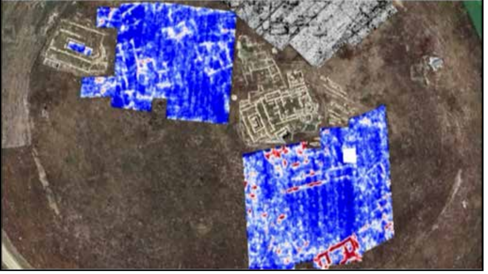
Resim 1: Merkezî Kilise'nin kuzey ve batısındaki alanlarda 2022, 2023 ve 2024 sezonlarında gerçekleştirilen yer radarı çalışmalarının sonuçları.
