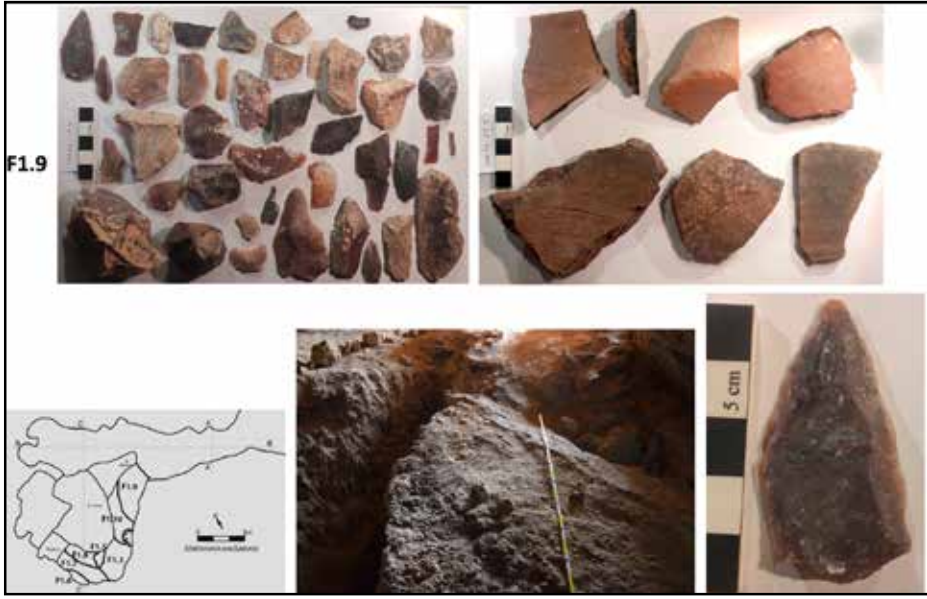
Resim 5: F1-9 birimindeki sertleşmiş dolgu (alt ortada), Levallois uç (alt sağ), yontma taşlar (üst sol) ve seramikler (üst sağda).
