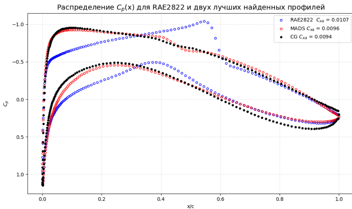
Рисунок 11. Распределения C_p(x) оптимумов и RAE2822
