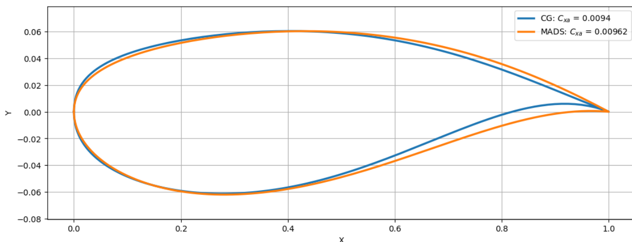
Рисунок 10. Найденные локальные оптимумы с наименьшим сопротивлением
