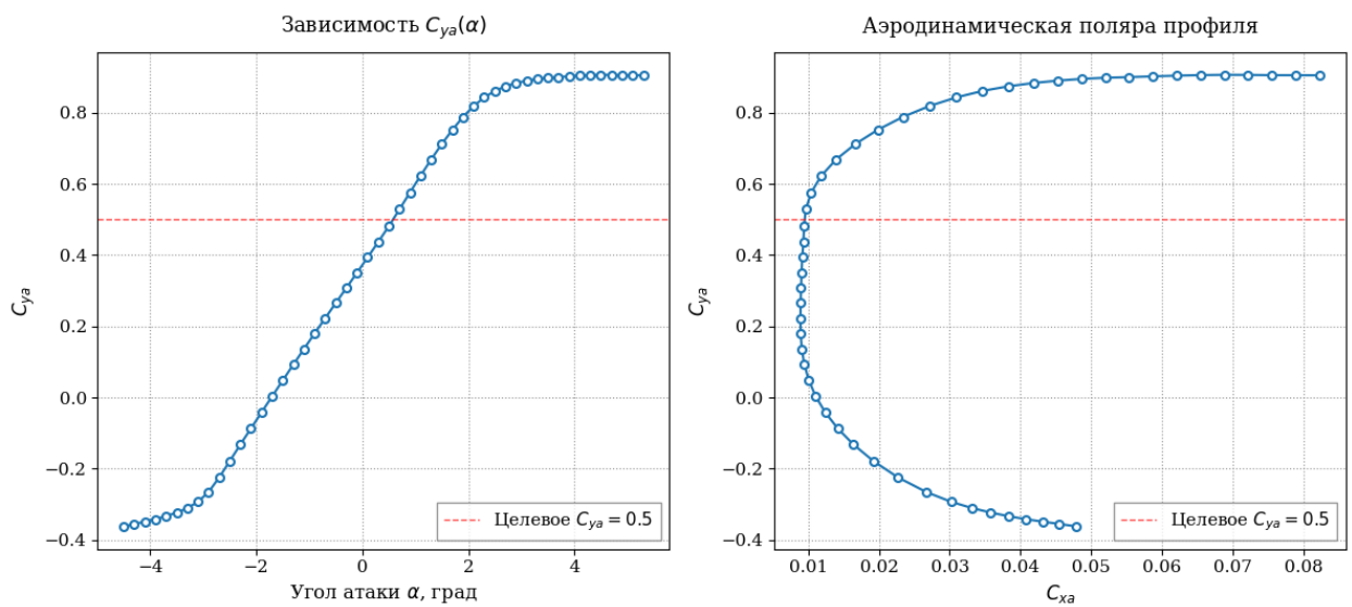
Рисунок 13. Интегральные характеристики полученного профиля
