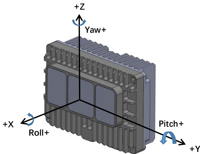
图11 E1R 激光雷达坐标系定义
