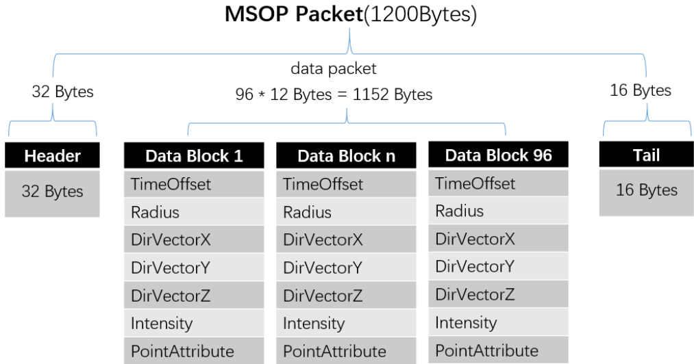
图12 MSOP Packet 数据包定义示意图
