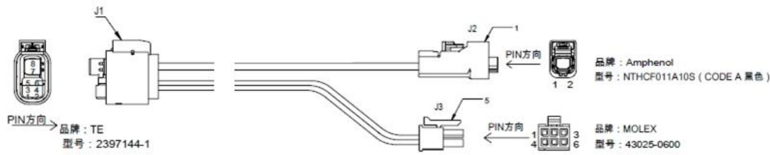
图8 车载以太网电源线束
