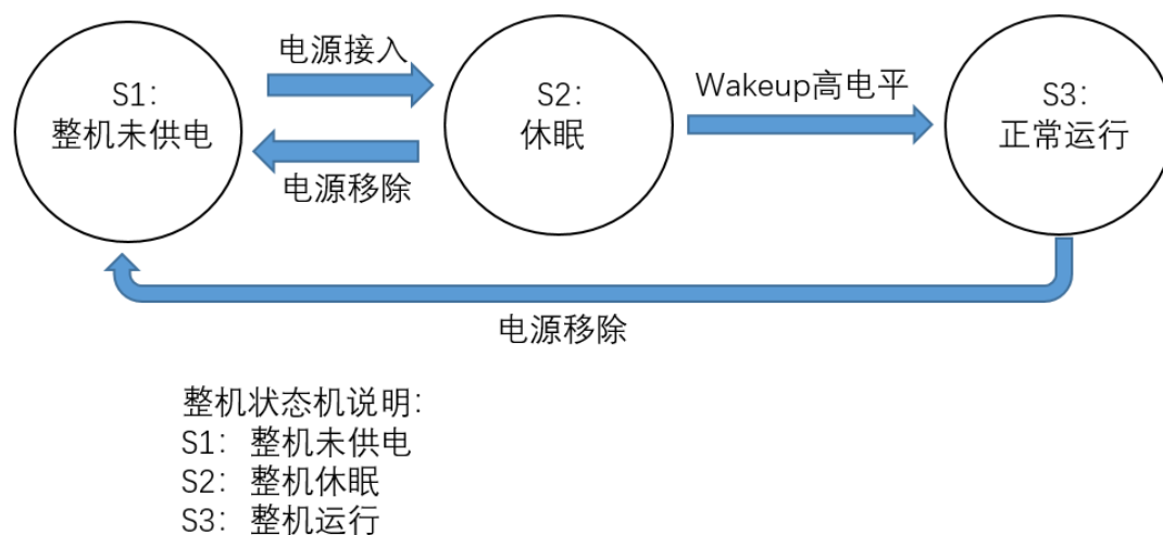
图9 激光雷达状态机描述
