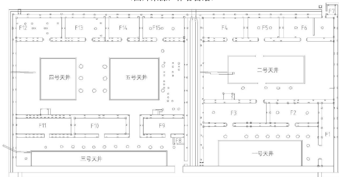
图 6.31 中央官署遗址平面 (图片来源: 作者自绘)
