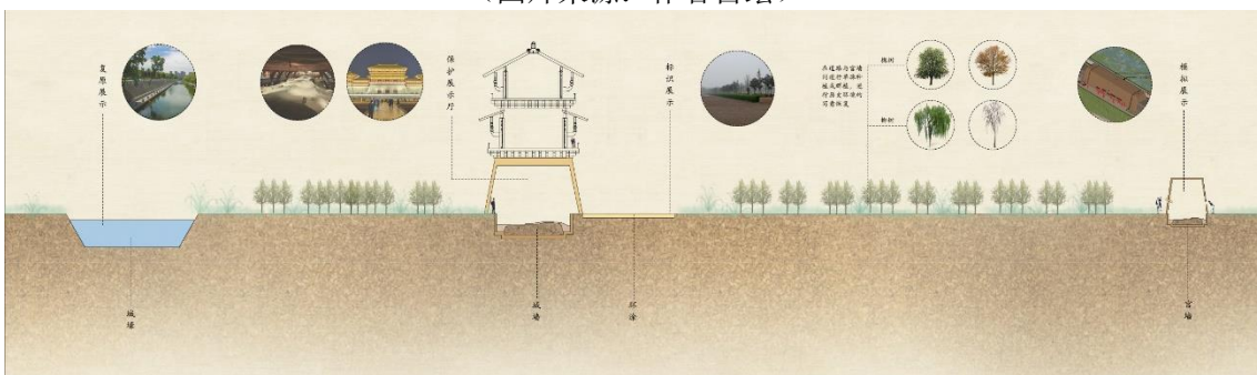
图 6.39 西安门展示节点剖面图 (图片来源: 作者自绘)
