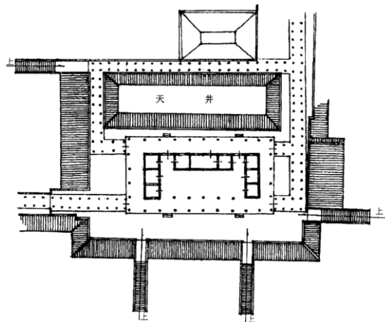
图 6.26 椒房殿台上复原平面图（图片来源：杨鸿勋宫殿考古通论）
