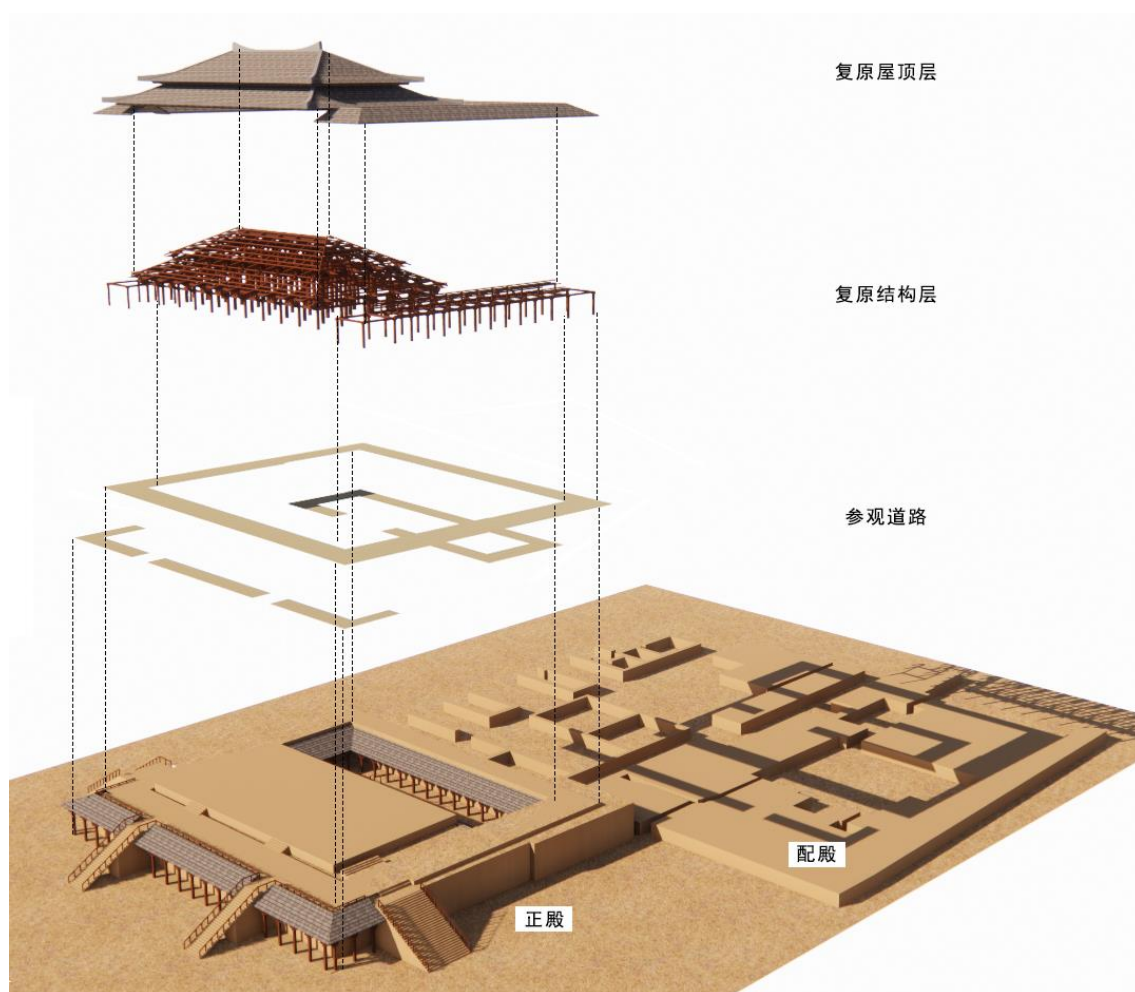
图 6.28 椒房殿遗址展示解析 (图片来源：作者自绘)
