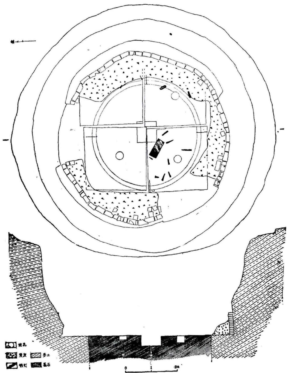
图 2-9 明堂中心柱柱坑平、剖面图 1
