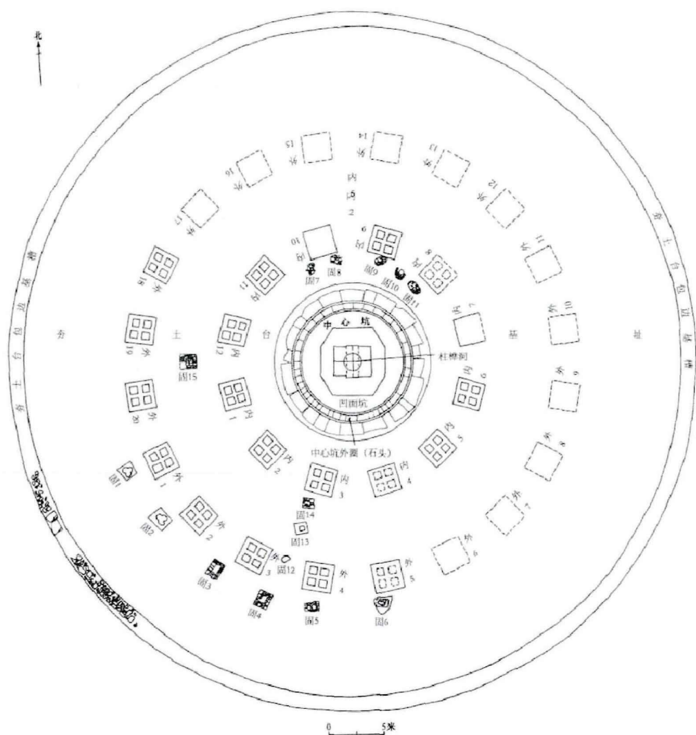
图 2-13 天堂遗址遗迹实测图 1
