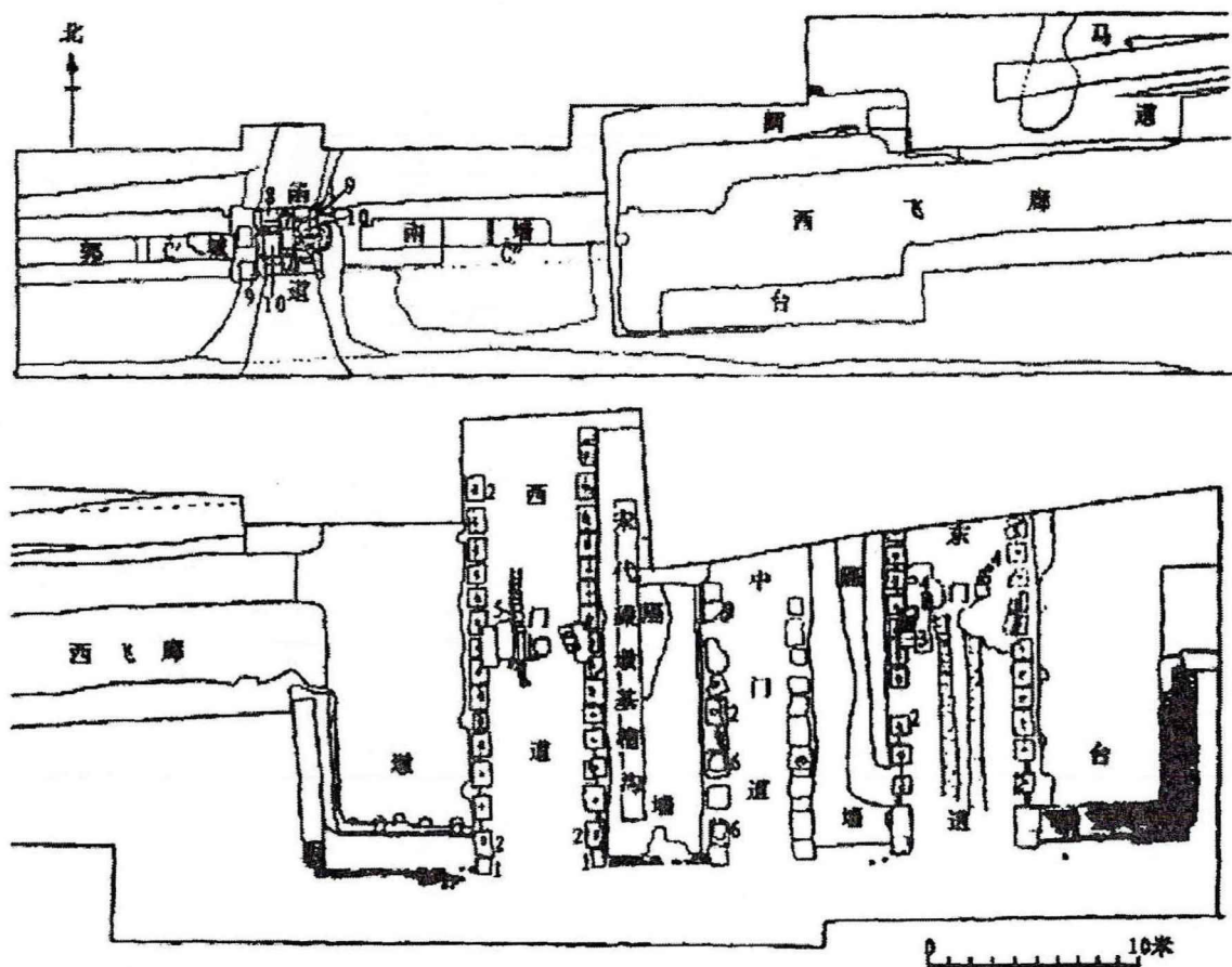
图 2-1 盛唐前期定鼎门遗址平面图 1
