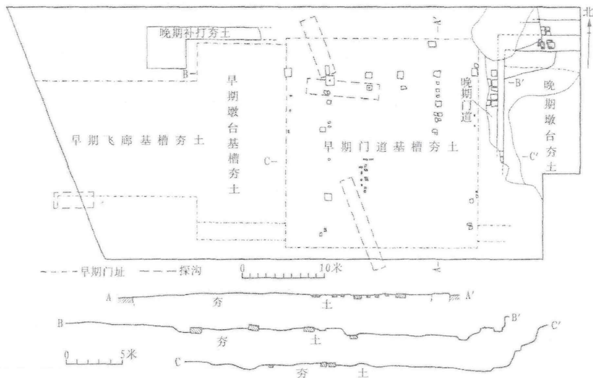
图 2-5 应天门遗址 2001~2002 发掘平、剖面图 1
