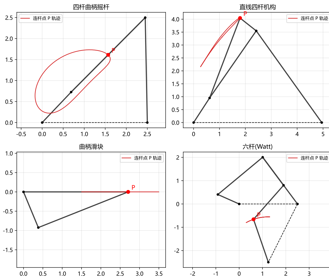
图 3: 四类基准机构 (黑色为机构, 红色为连杆点 P 轨迹)
