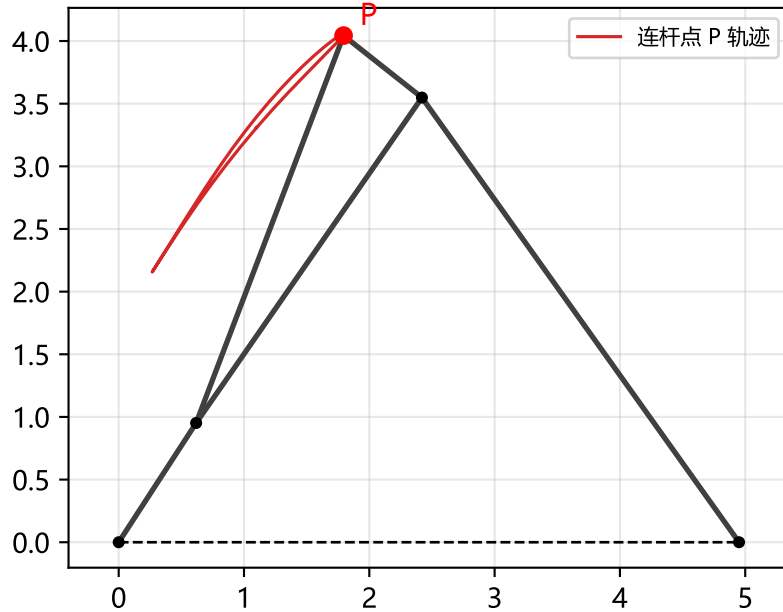
六杆(Watt)
