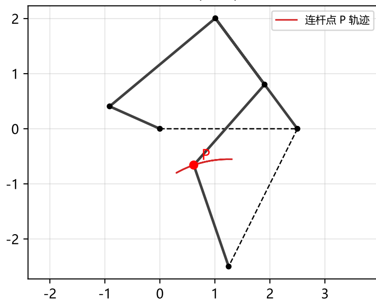
六杆(Watt)
