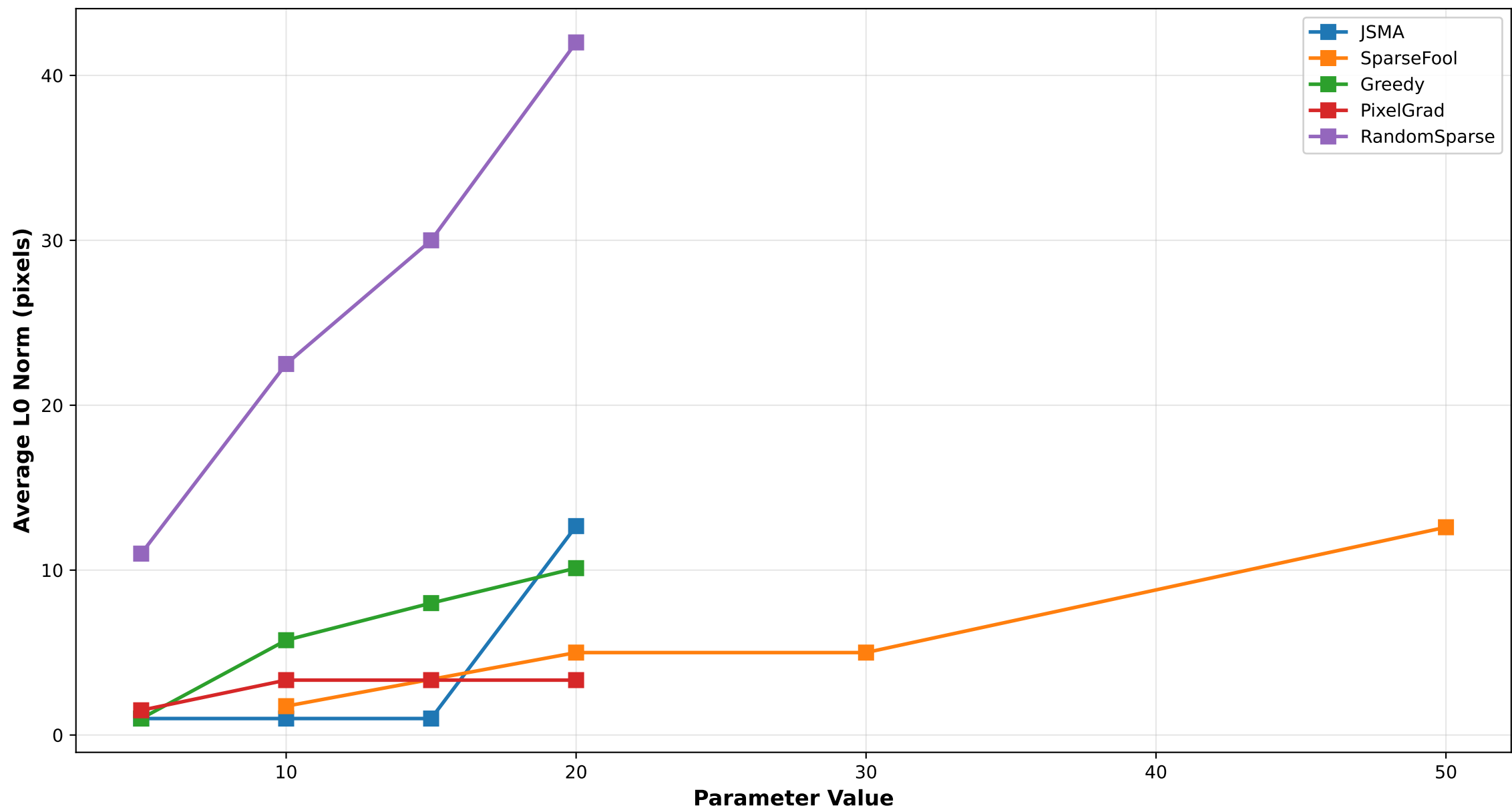
Parameter Sensitivity: L0 Norm vs Parameter Value
