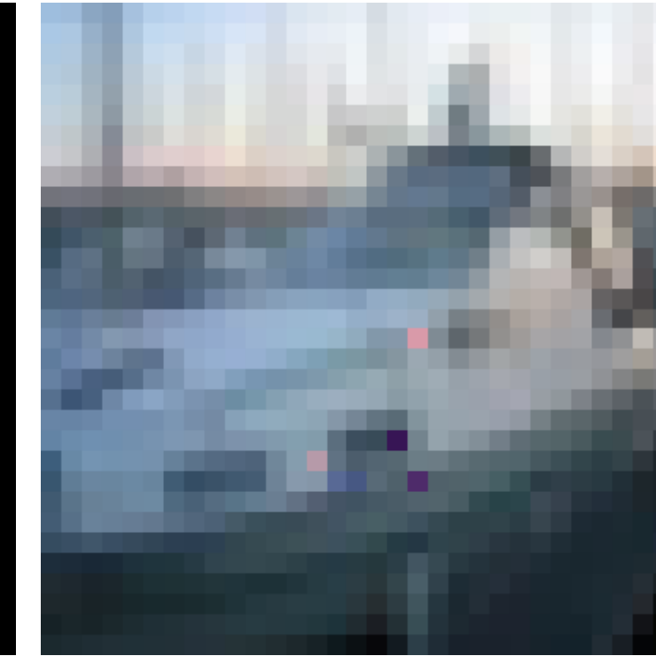
SparseFool → automobile
