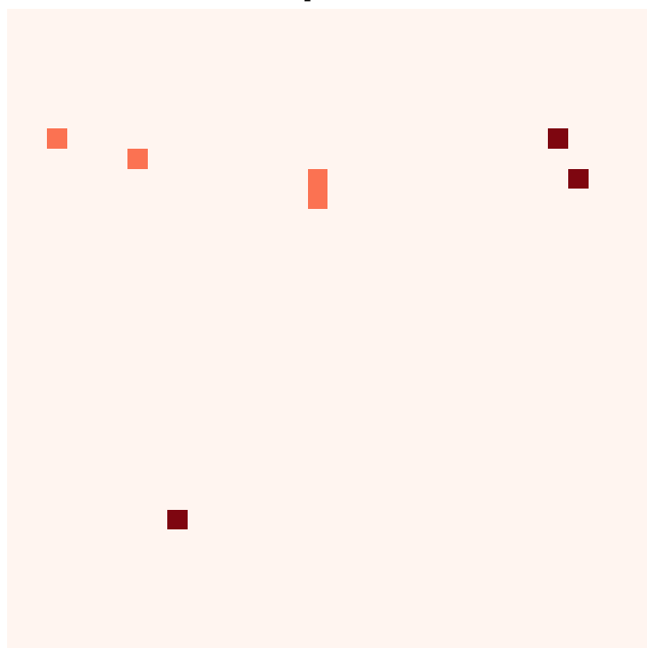
JSMA 10 pixels
