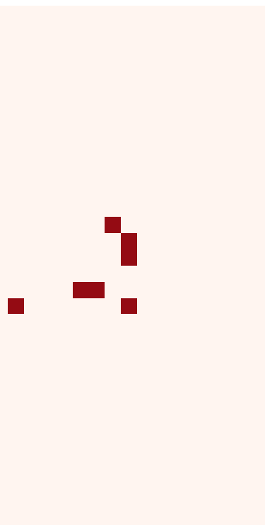
JSMA 7 pixels
