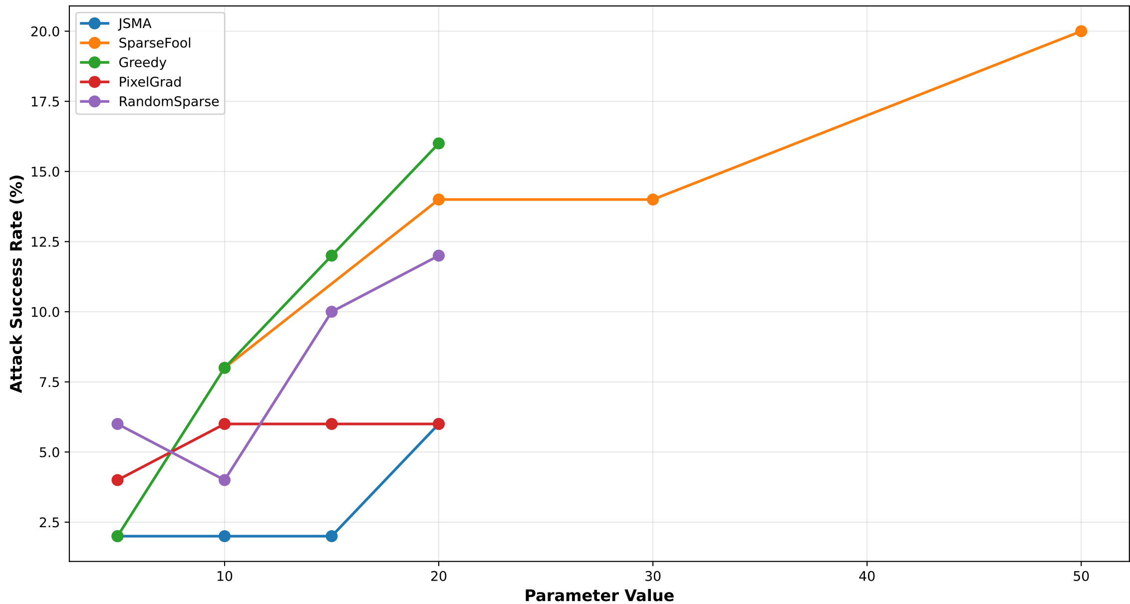
Parameter Sensitivity: ASR vs Parameter Value
