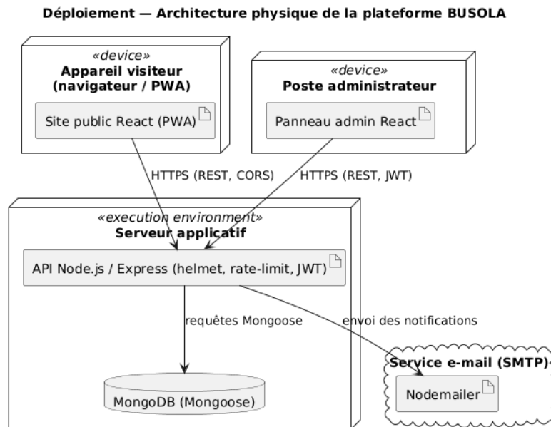
Figure 8 : Déploiement de la plateforme BUSOLA
