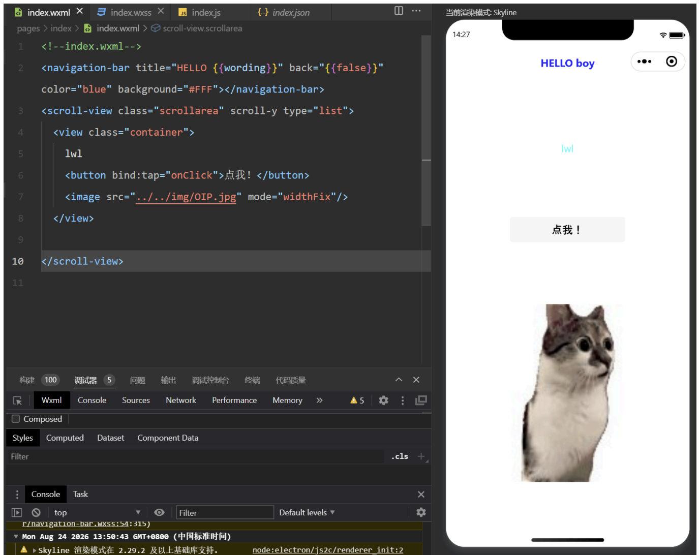
图 1 WXML 页面结构及运行效果
