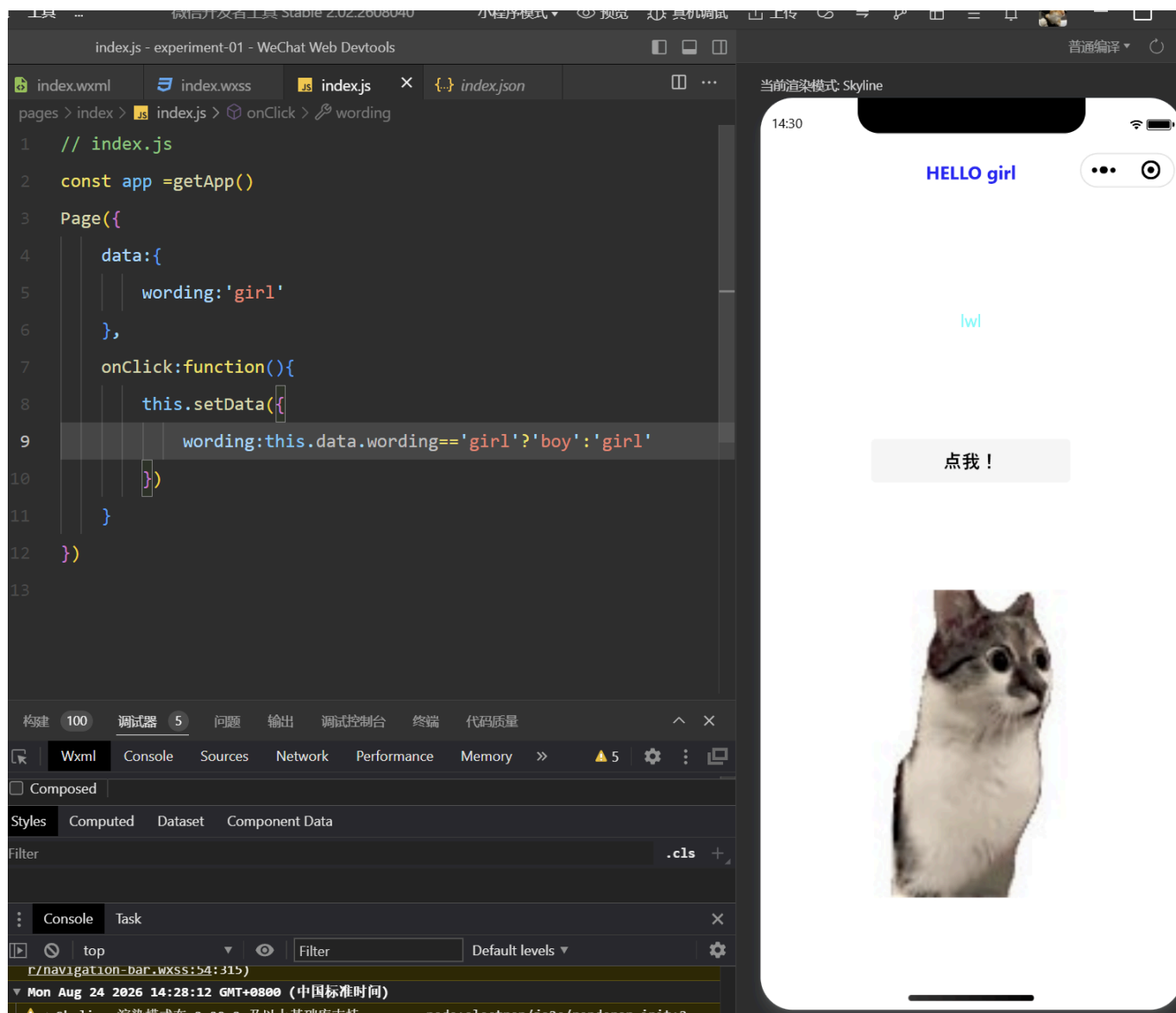
图2 JavaScript 中的标题切换代码
