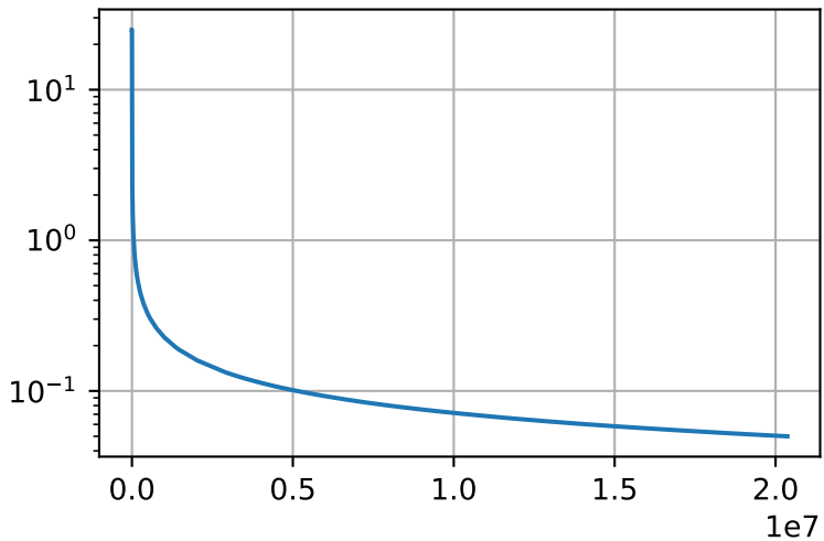
\Delta_t
