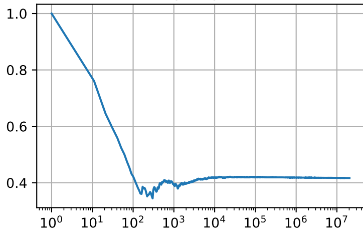
N_t^\omega
