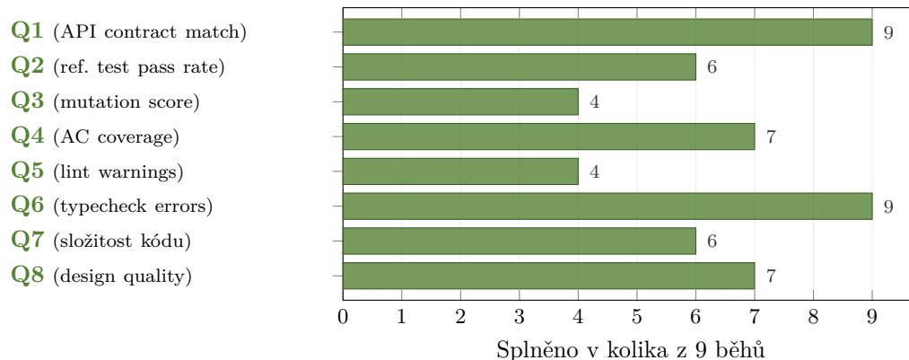
Obrázek 5.2: Míra splnění operačních prahů produktové metriky (Q1–Q8) napříč devíti běhy ( Q2 \geq 37 , Q3 \geq 70\% , Q4 \geq 24 , Q5 \leq 1 , Q7 \leq 1 ; viz sekce 3.1.3). Striktní exit z tabulky 3.10 ( Q2 = 42/42 , Q5 = 0 , Q7 = 0 porušení) nesplnil žádný běh. Q1 a Q6 byly splněny ve všech bězích; Q3 a Q5 nejméně často. Q3 počítáno ze 7 běhů (2 bez dat). Metriky efektivity (E1–E3) nemají exit kritérium a nejsou zahrnuty.
