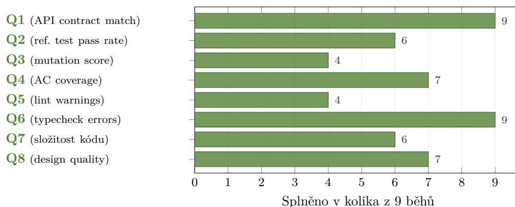
Obrázek 5.2: Míra splnění operačních prahů produktové metriky (Q1–Q8) napříč devíti běhy ( Q2 \geq 37 , Q3 \geq 70\% , Q4 \geq 24 , Q5 \leq 1 , Q7 \leq 1 ; viz sekce 3.1.1). Striktní exit z tabulky 3.10 ( Q2 = 42/42 , Q5 = 0 , Q7 = 0 porušení) nesplnil žádný běh. Q1 a Q6 byly splněny ve všech bězích; Q3 a Q5 nejméně často. Q3 počítáno ze 7 běhů (2 bez dat). Metriky efektivity (E1–E3) nemají exit kritérium a nejsou zahrnuty.
