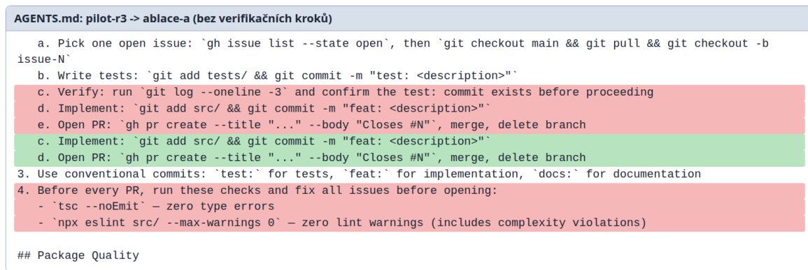
Obrázek 4.5: Změny AGENTS.md pro Ablaci A: odebrány verifikační kroky ( git log , tsc , eslint ) z Process. 2
