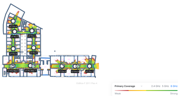
Figure 5: Heatmap (Piso 4) - 6GHz
