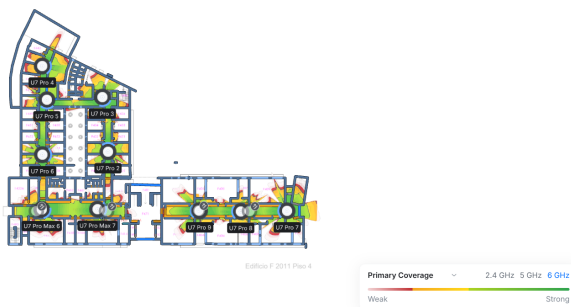
Figure 5: Heatmap (Piso 4) - 6GHz
