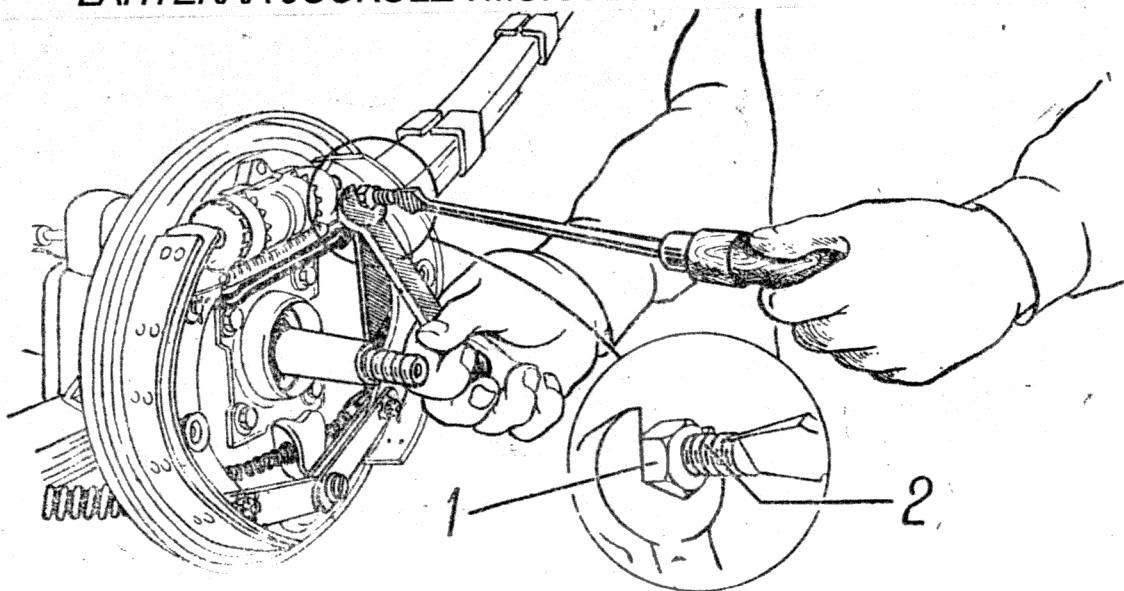
Рис. 25 — Регулировка положения разжимных рычагов тормозных колодок.
