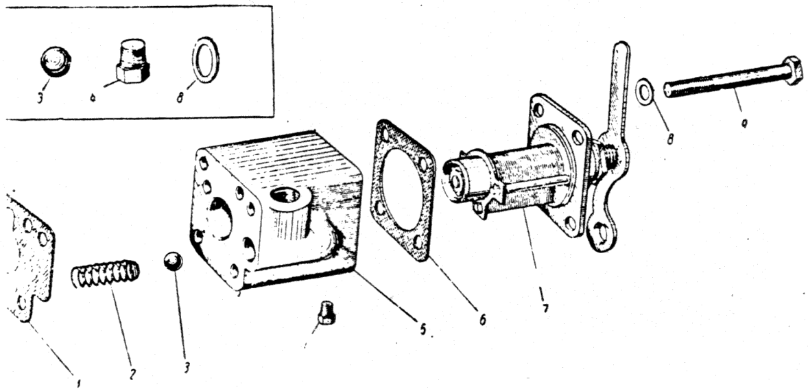
Фиг. 23. Фильтр грубой очистки масла.
