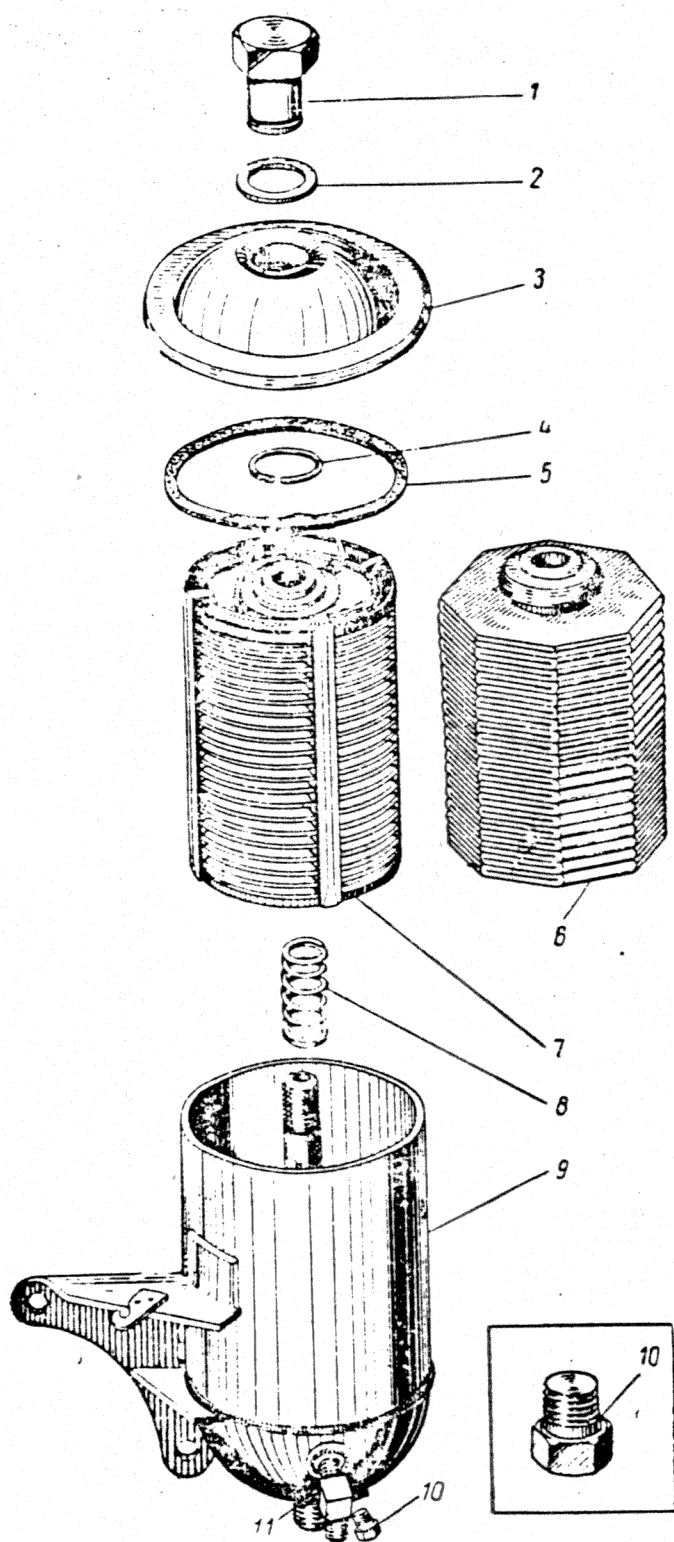
Фиг. 26. Фильтр тонкой очистки масла.
