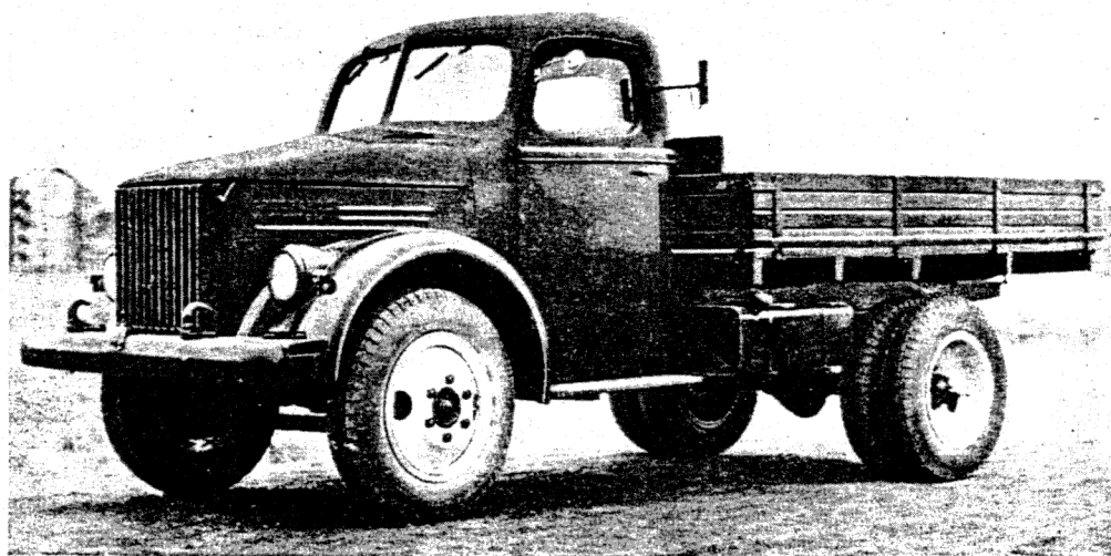
Gaz 3 t. kuorma-auto, 70 hv. 2800 k./min.
