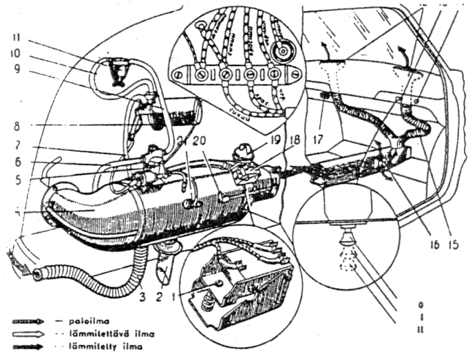
JALTAN lämmityslaitte.
