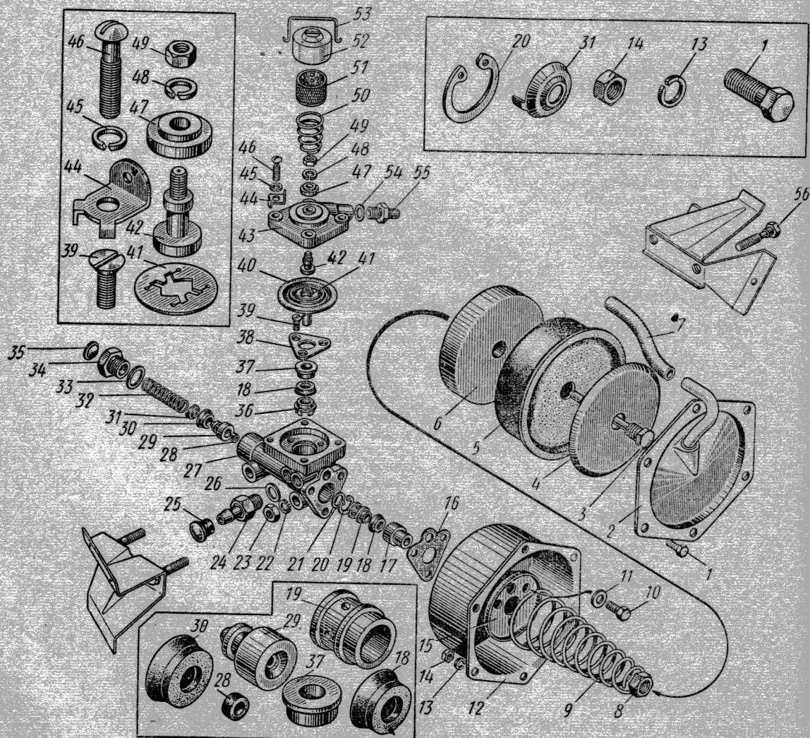
Рис. 68. Гидровакуумный усилитель тормоза
