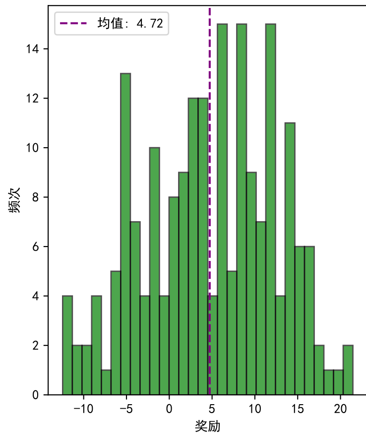
总奖励分布
