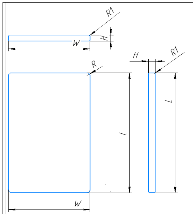
Рисунок 2.1 – Модель столешницы с обозначением размеров ( L , H , W , R , R1 ).
