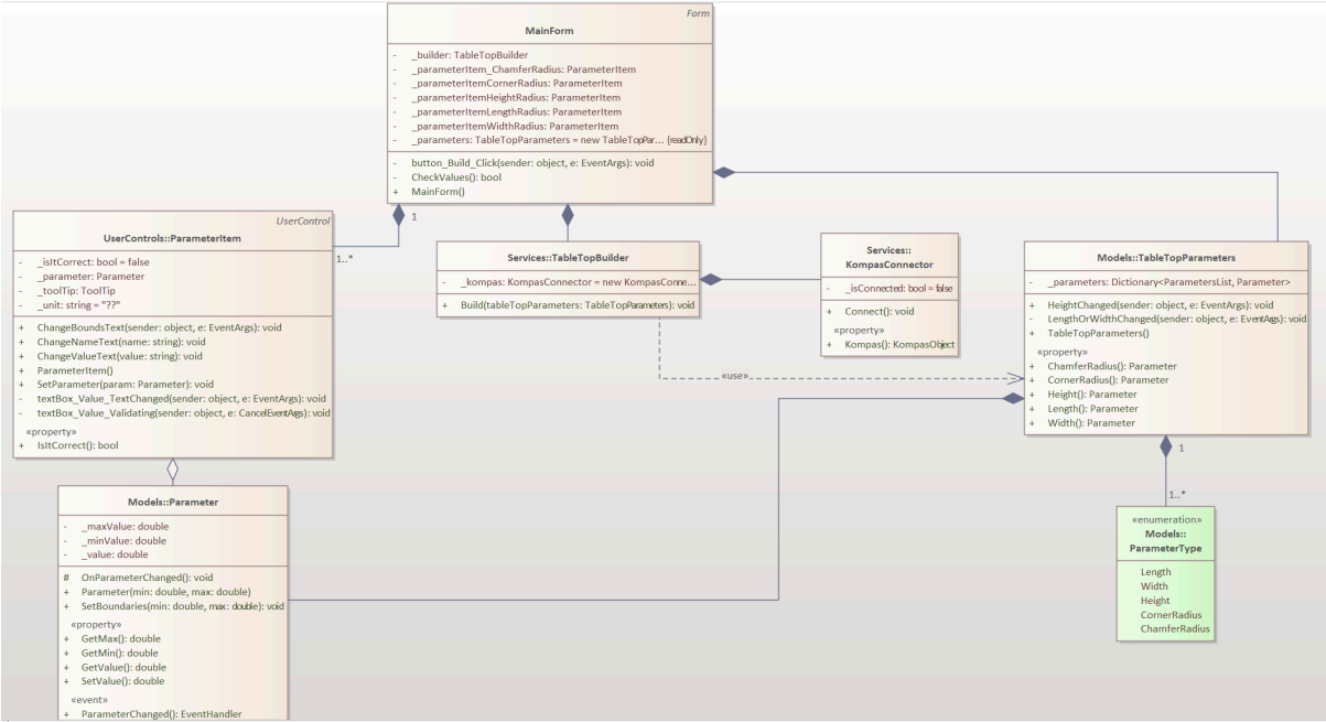
Рисунок 3.1 – UML-диаграмма классов плагина «Столешница».
