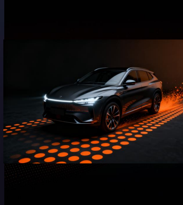
Hidream
