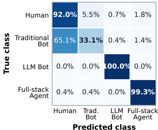
(d) Quadbot - CBAF-Net
