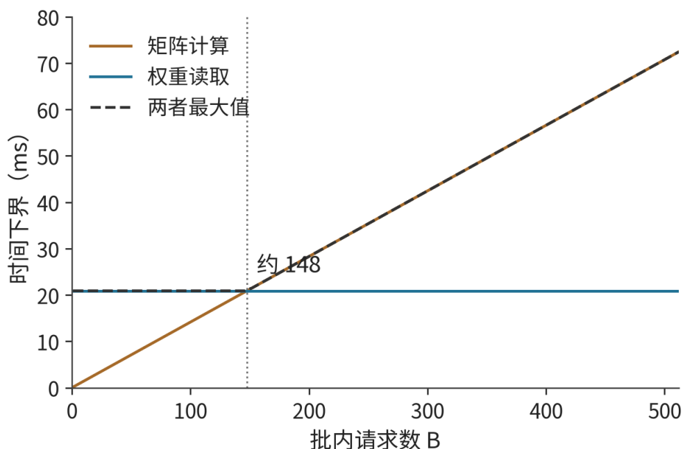
图 1-11 批内请求增加时，矩阵运算量按 2BN 增长，权重读取保持每批 70 GB。约 148 个请求处两项下界相等，随后计算耗时决定整体速度。
