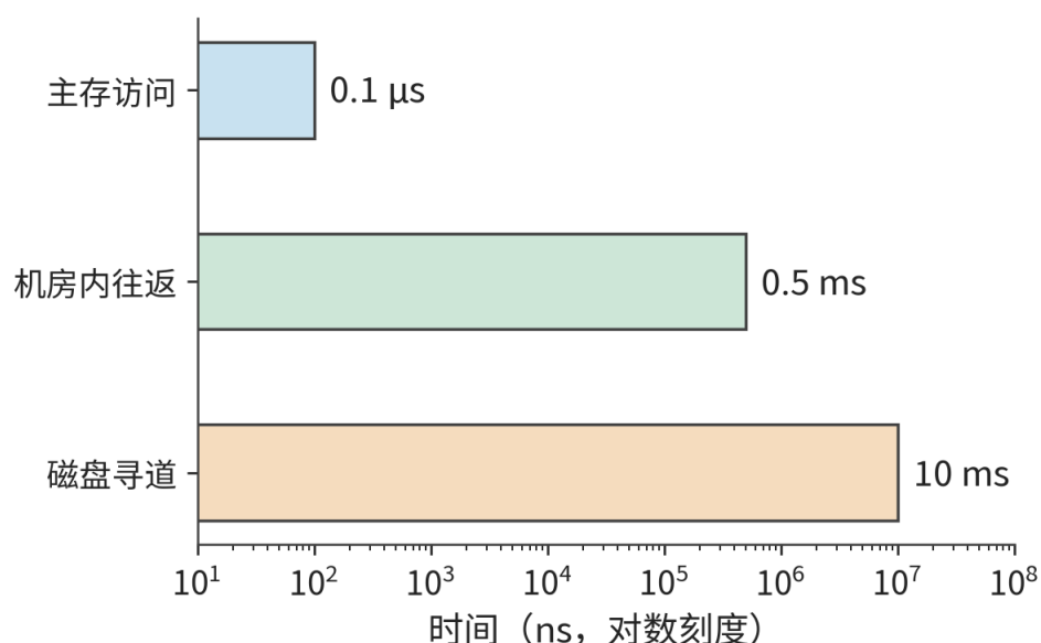
图 1-6 Jeff Dean 2009 年演讲中的三种操作延迟。横轴为对数刻度，每相邻数量级相差十倍；先识别操作，再比较它们在串行等待中的代价。
