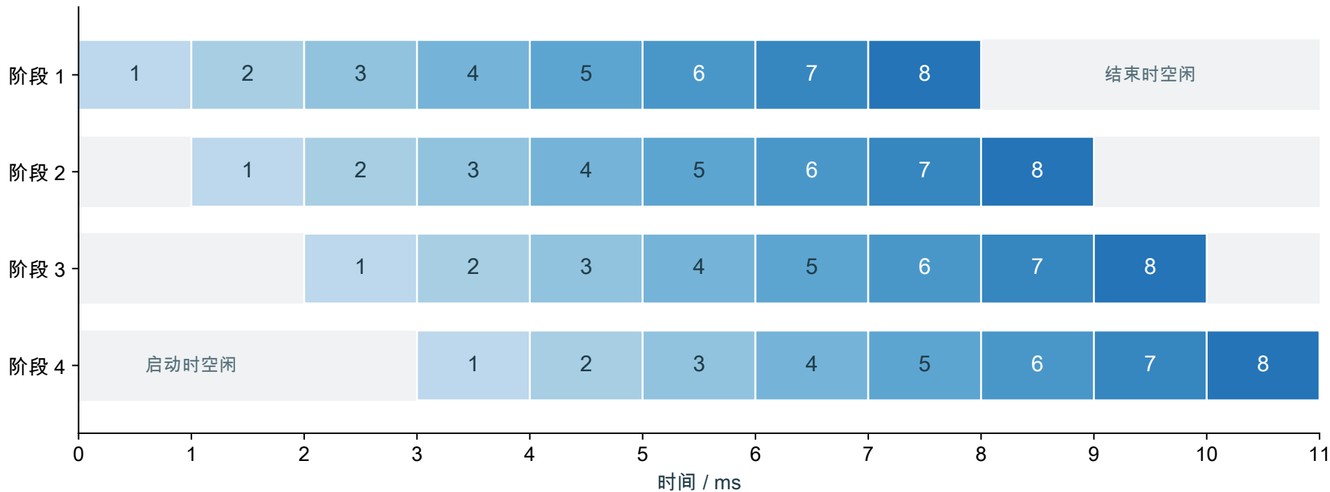
同一微批依次通过四个阶段；不同微批可以同时计算
