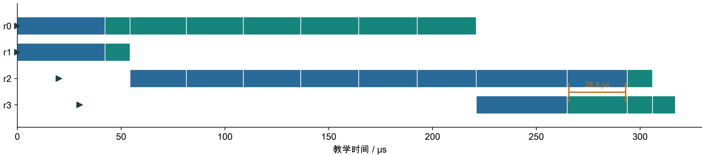
Decode 优先分块〔教学〕 · 总时间 317 \mu\text{s} , 最大间隔 29 \mu\text{s}
