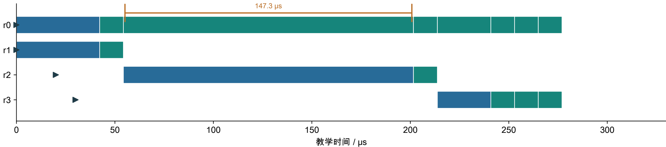
连续批处理〔教学〕 · 总时间 277 \mu\text{s} , 最大间隔 147 \mu\text{s}
