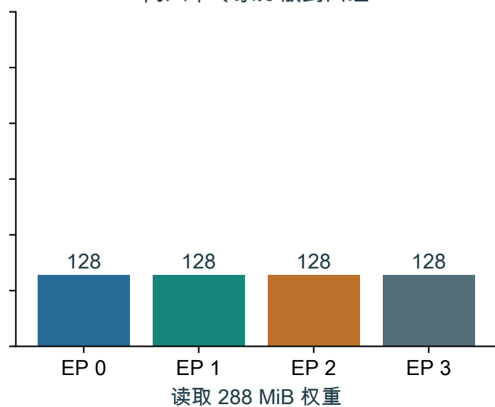
同八个专家分散到四组
