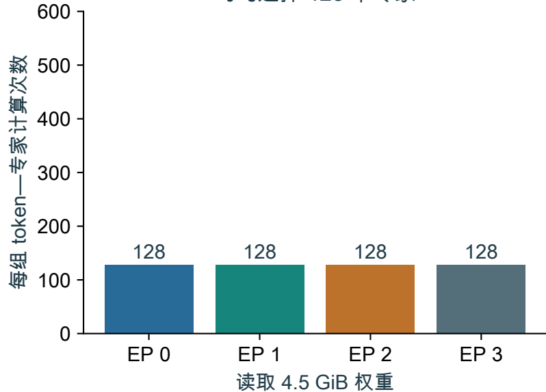
均匀选择 128 个专家
