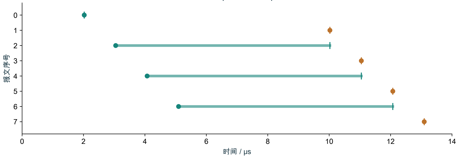
传播时延为 1/9\ \mu\text{s} : 约 13.1\ \mu\text{s} 全部交付
