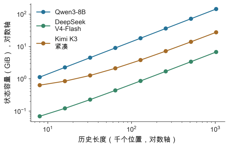
图 2-18 历史增长时的状态容量。横纵轴均为对数刻度；Qwen 逐位置追加 KV，Kimi K3 紧凑表示包含固定递推状态和增长的 MLA 历史，DeepSeek V4-Flash 按压缩块增加条目。
