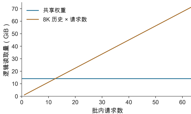
图 2-8 同一批次的主要投影权重可共享读取，各请求则各有一份历史。图中固定每请求 8K 历史，分别累计共享权重与独立 KV 的逻辑读取量。
