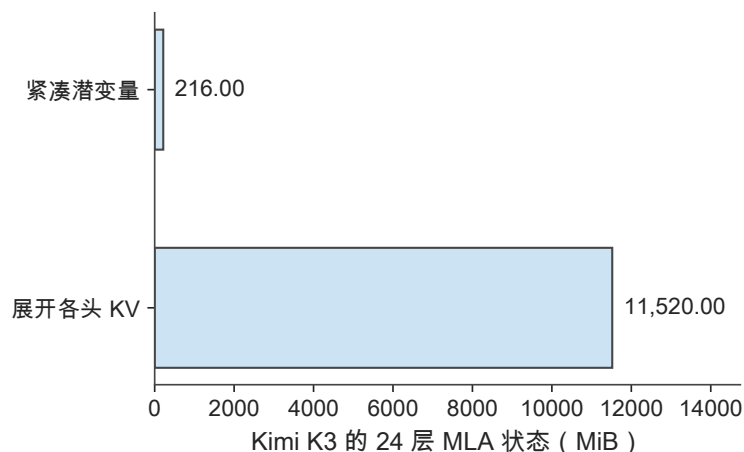
图 2-12 Kimi K3 的 24 层 MLA 在相同 8K 历史、BF16 下的两种保存量。紧凑路径保存上投影前的表示，展开路径保存各头的键和值。
