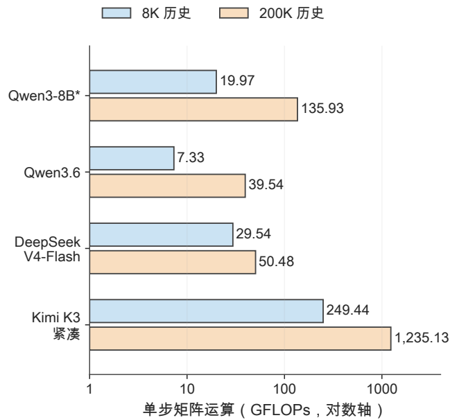
图 2-28 已有 8K / 200K 历史后再处理一个 token 的矩阵运算量。蓝、橙分别对应两种历史长度，横轴为对数刻度，柱端标出 GFLOPs。沿用表 2-C 的 decode 路径，Kimi K3 的 KDA 使用递推、MLA 使用紧凑表示。星号表示 Qwen3-8B 的 200K 条件超过本章固定配置的未缩放上下文上限，仅按原结构外推。
