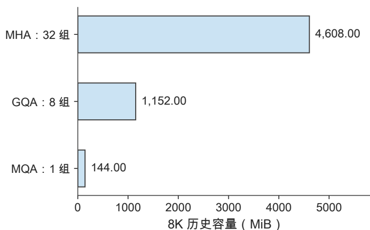
图 2-10 固定 Qwen 层数、头宽、8192 个历史位置与 BF16，只改变 KV 组数。实际模型采用 GQA；其余两柱是用于分析共享比例的结构变体。
