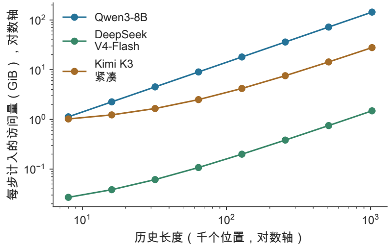
图 2-19 同一组模型每步计入的状态访问。逐位置历史计读取，递推矩阵计一读一写；这些是指定路径的逻辑数据量，用于比较容量与访问的不同增长方式。
