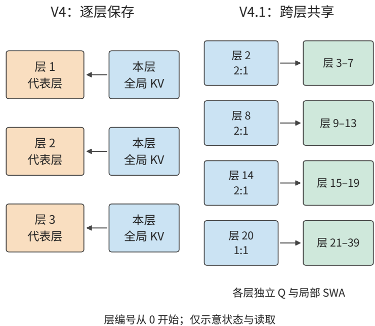
图 2-21 V4 与 V4.1 的全局 KV 保存方式。左侧以三个代表层示意逐层保存；右侧显示 V4.1 四个全局 KV 拥有层及共享关系。实线表示数据读取；各使用层仍有自己的 Q 与局部 SWA，图中省略其他计算。
