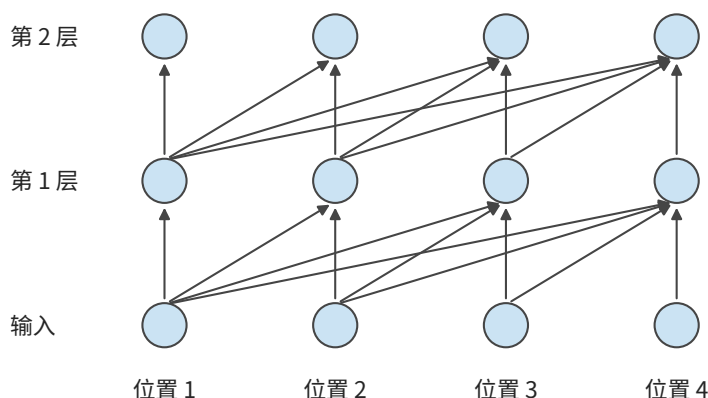
图 2-2 因果 Transformer 的层间依赖。各查询读取上一层中允许访问的位置；上一层完成后，同一层的已知输入位置可以并行计算。
