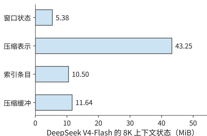
图 2-14 DeepSeek V4-Flash 在 8K 上下文下的四项状态。窗口、压缩上下文和索引是已保留的上下文；压缩缓冲保存尚在汇总或更新中的数据，单独计入容量。
