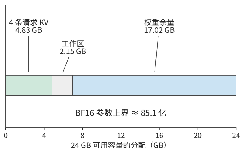
图 2-34 从设备反推权重预算。24 GB 中先保留 4 条 8K 请求的 KV 和 2 GiB 工作区，余量给出 BF16 参数上界；图中容量均为十进制 GB。
