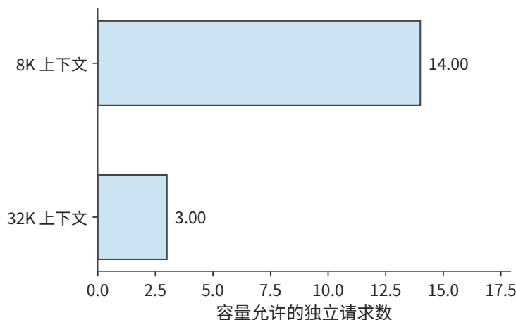
图 2-33 70B 的 4-bit 方案在同一张 80 GB 设备上，上下文长度从 8K 增至 32K 时允许保留的独立请求数。每请求状态增加，使剩余空间容纳的请求数减少。
