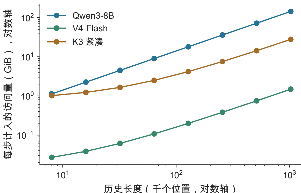
图 2-19 同一组模型每步计入的状态访问。逐位置历史计读取，递推矩阵计一读写；这些是指定路径的逻辑数据量，用于比较容量与访问的不同增长方式。
