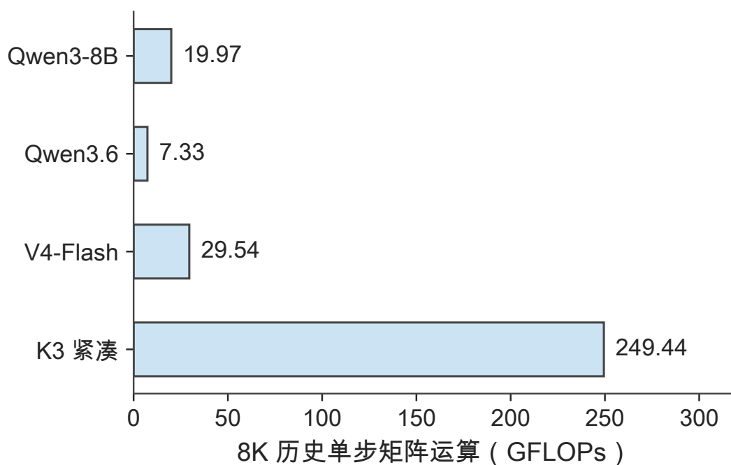
图 2-26 相同单请求、已有 8K 历史时的单步矩阵运算量。按各模型在表 2-C 说明的执行路径累计，K3 采用紧凑 MLA。
