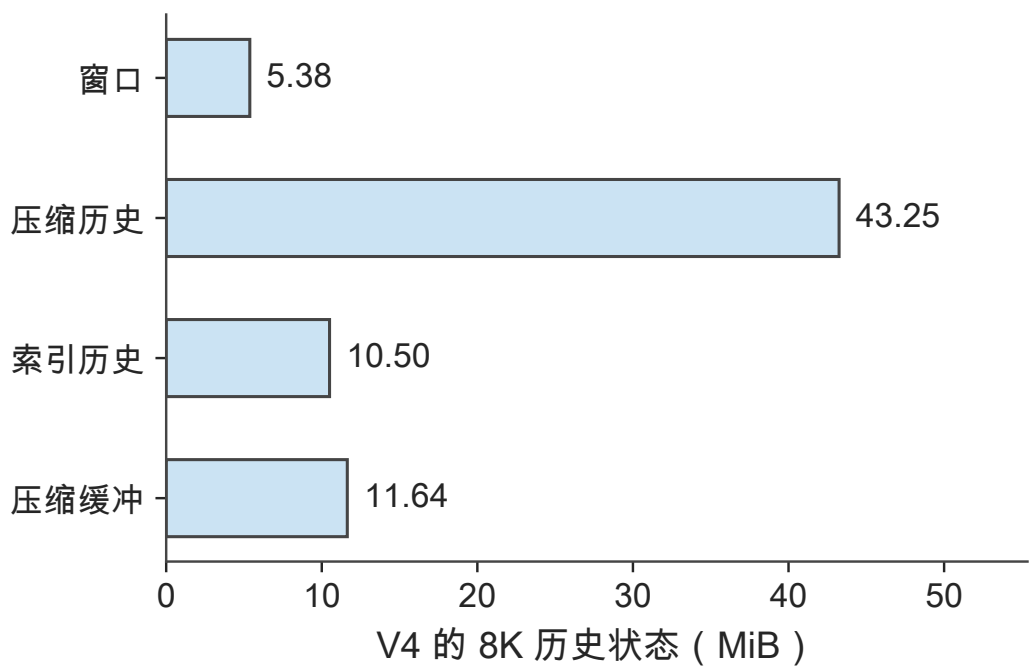
图 2-14 V4 在 8K 历史下的四项状态。窗口、压缩历史和索引是已保留的历史；压缩缓冲保存尚在汇总或更新中的数据，单独计入容量。
