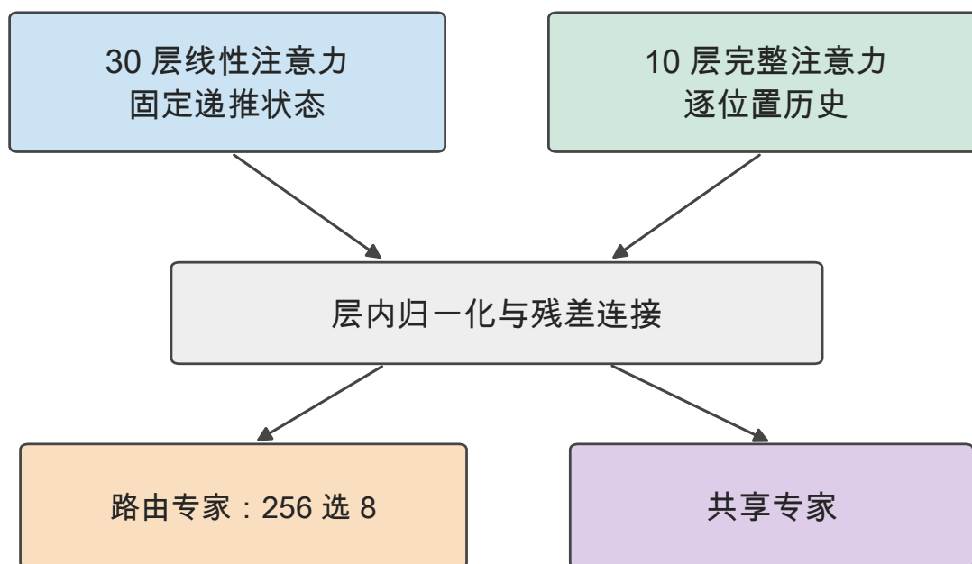
图 2-17 Qwen3.6 的两类层。配置决定每层采用线性或完整注意力，随后都执行路由专家和共享专家；上方分支表示层型，模型分别有 30 层与 10 层。
