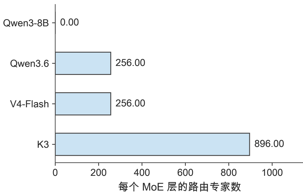
图 2-24 每个 MoE 层保存的路由专家数量。Qwen3-8B 使用稠密前馈层，其路由专家数为零；每个 token 实际选中数见表 2-A。
