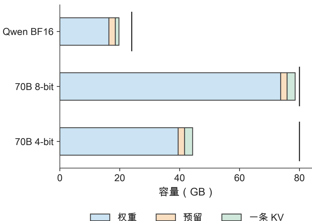
图 2-29 权重、固定预留和一条请求 KV 的逐项容量。短竖线标出各设备容量；KV 采用 BF16、历史长度 8192，固定预留为 2 GiB。
