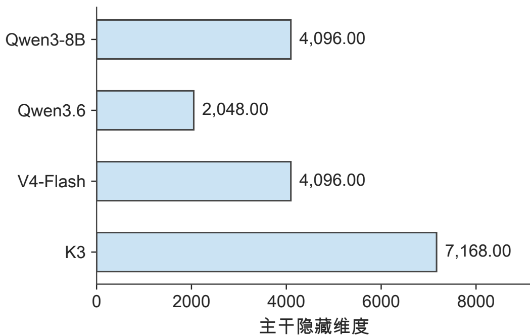
图 2-23 同一线性尺度下的主干隐藏维度。每个位置的特征宽度决定投影的输入或输出尺寸。
