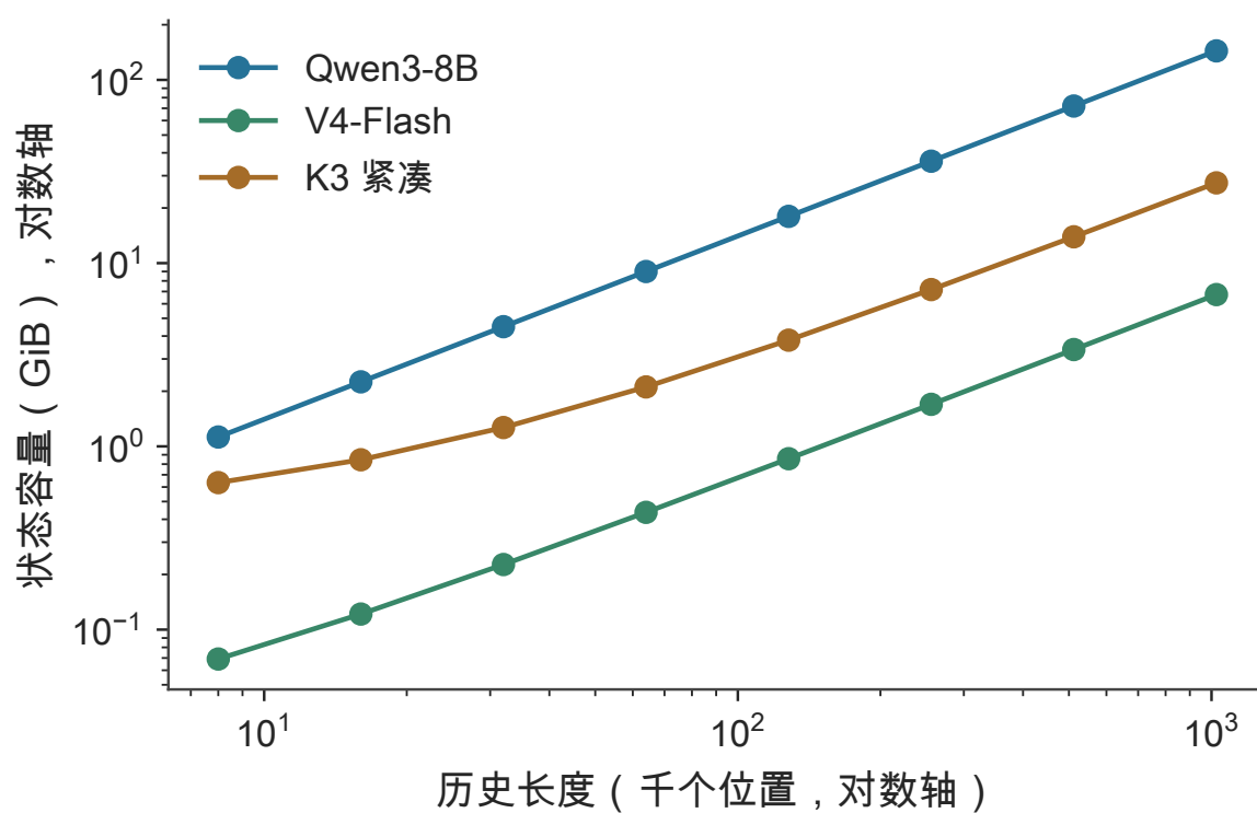
图 2-18 历史增长时的状态容量。横纵轴均为对数刻度；Qwen 逐位置追加 KV，K3 紧凑表示包含固定递推状态和增长的 MLA 历史，V4 按压缩块增加条目。
