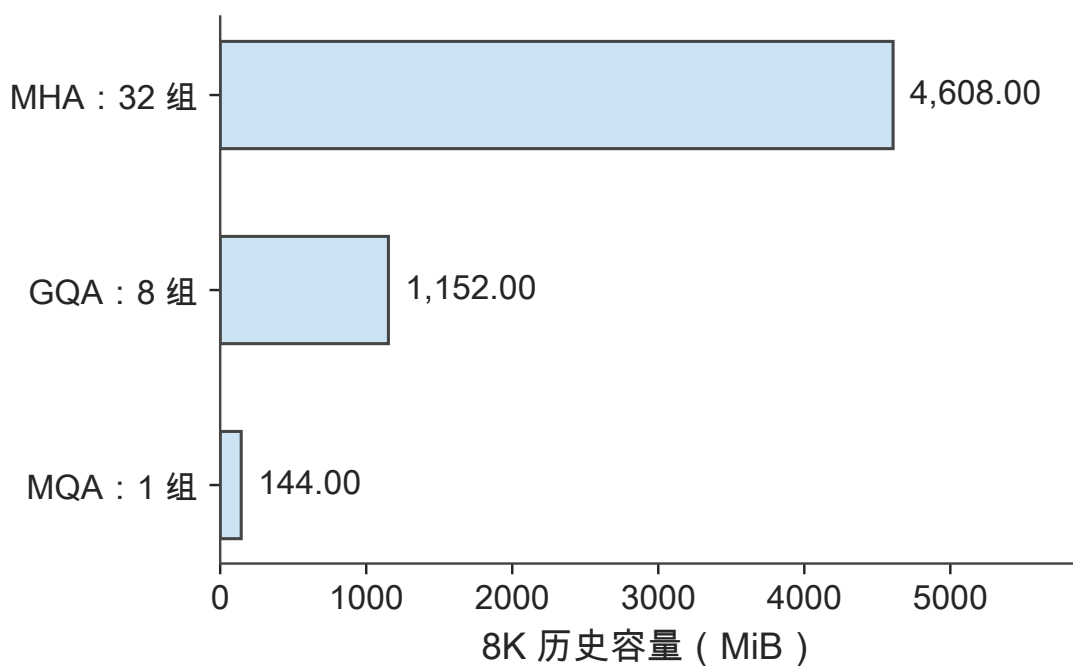
图 2-10 固定 Qwen 层数、头宽、8192 个历史位置与 BF16，只改变 KV 组数。实际模型采用 GQA；其余两柱是用于分析共享比例的结构变体。
