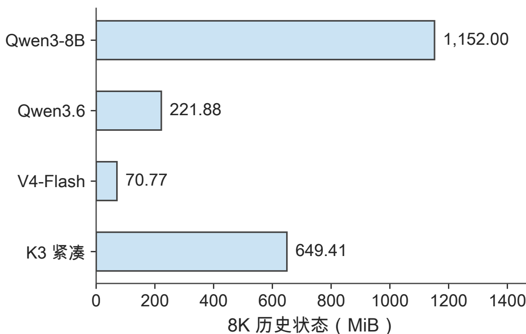
图 2-27 相同 8K 历史下的每请求状态。历史表示采用 BF16，递推矩阵和压缩缓冲采用相应实现的精度；各项合计对应表 2-C。
