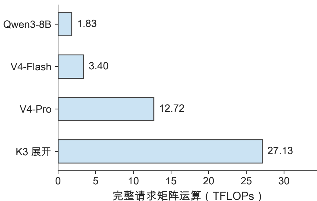
图 2-32 同一 128 输入、四输出请求的矩阵运算量。模型执行范围与缓存路径见本节题设；这是逐调用累计的计算量。
