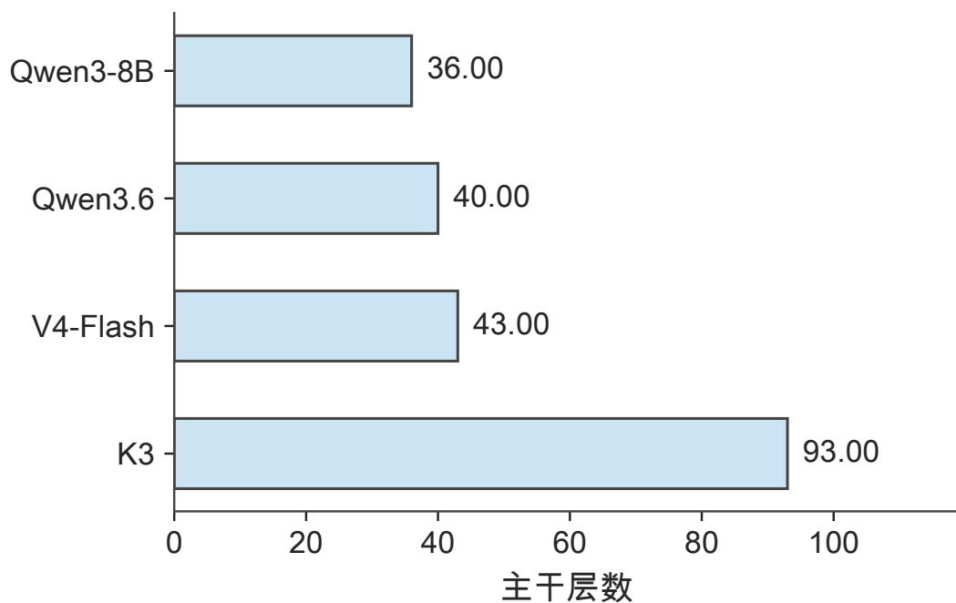
图 2-22 四模型的主干层数，使用同一线性尺度。层数决定同类工作沿网络深度重复多少次。
