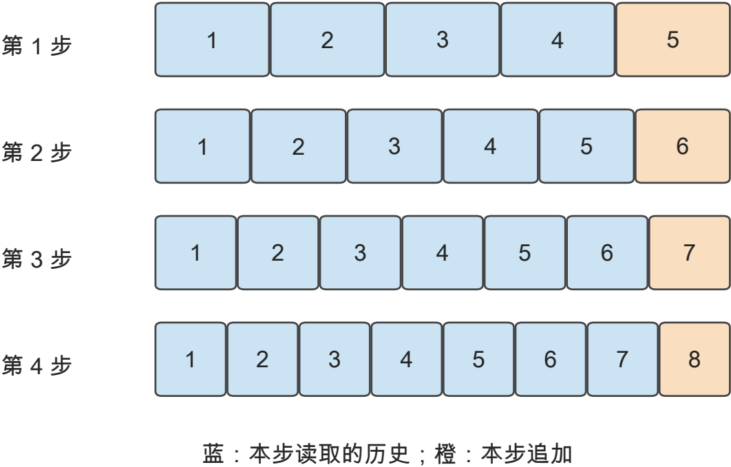
图 2-7 四步生成的历史读写。每一步读取蓝色的已有位置，再追加一个橙色新位置；本图初始历史为四，四步后保留八个位置。
