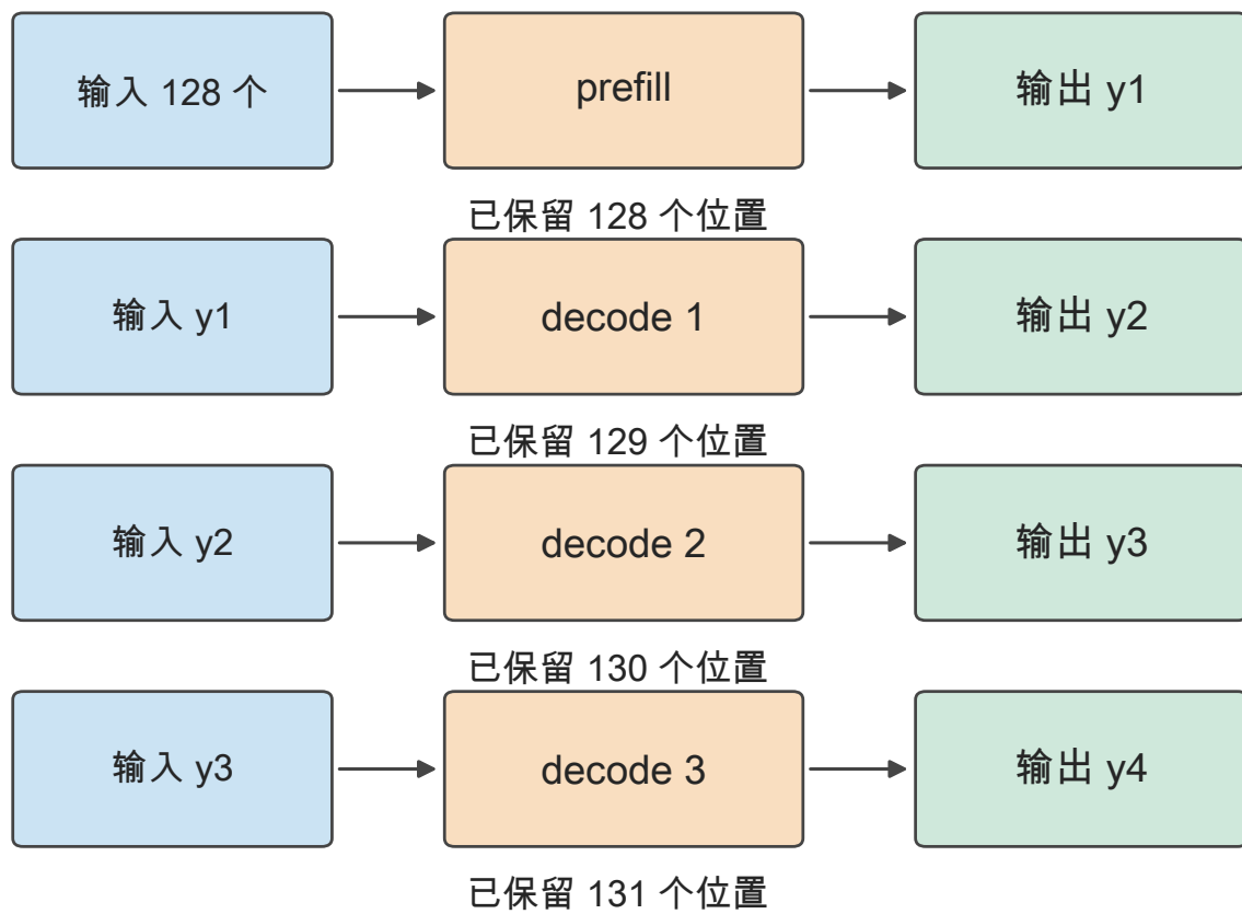
图 2-31 生成四个输出的调用顺序。prefill 处理 128 个输入并产生首输出，随后三次 decode 各将前一输出送回模型；最终保留 131 个位置。
