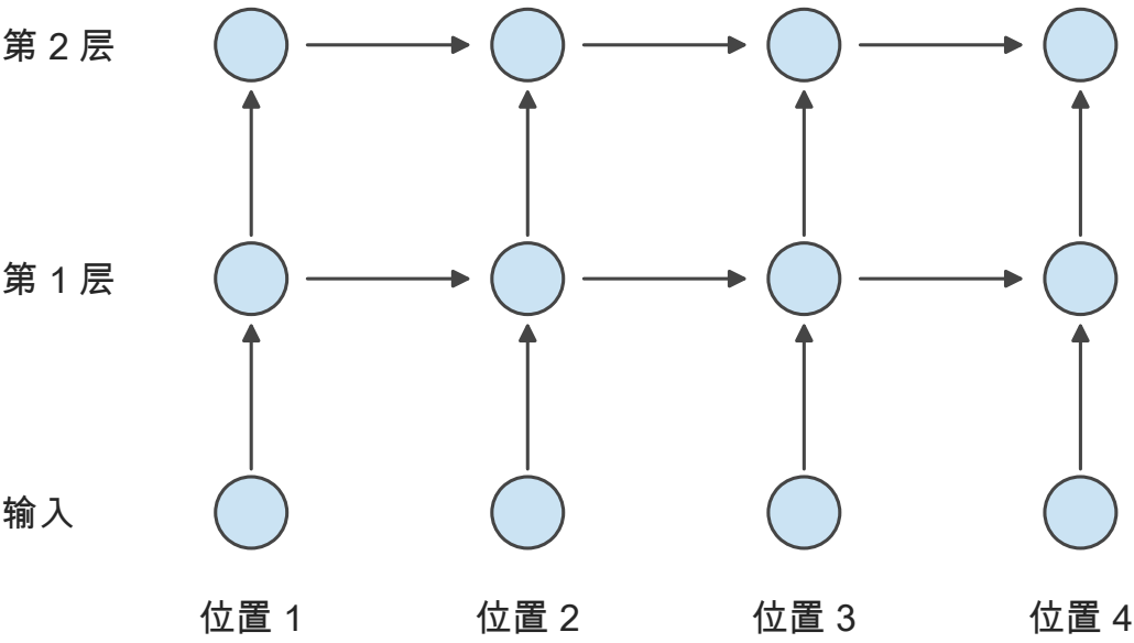
图 2-1 循环神经网络的依赖。相同颜色的圆点表示各位置的计算，箭头指向需要前一结果的节点；同层位置沿横向逐次推进。
