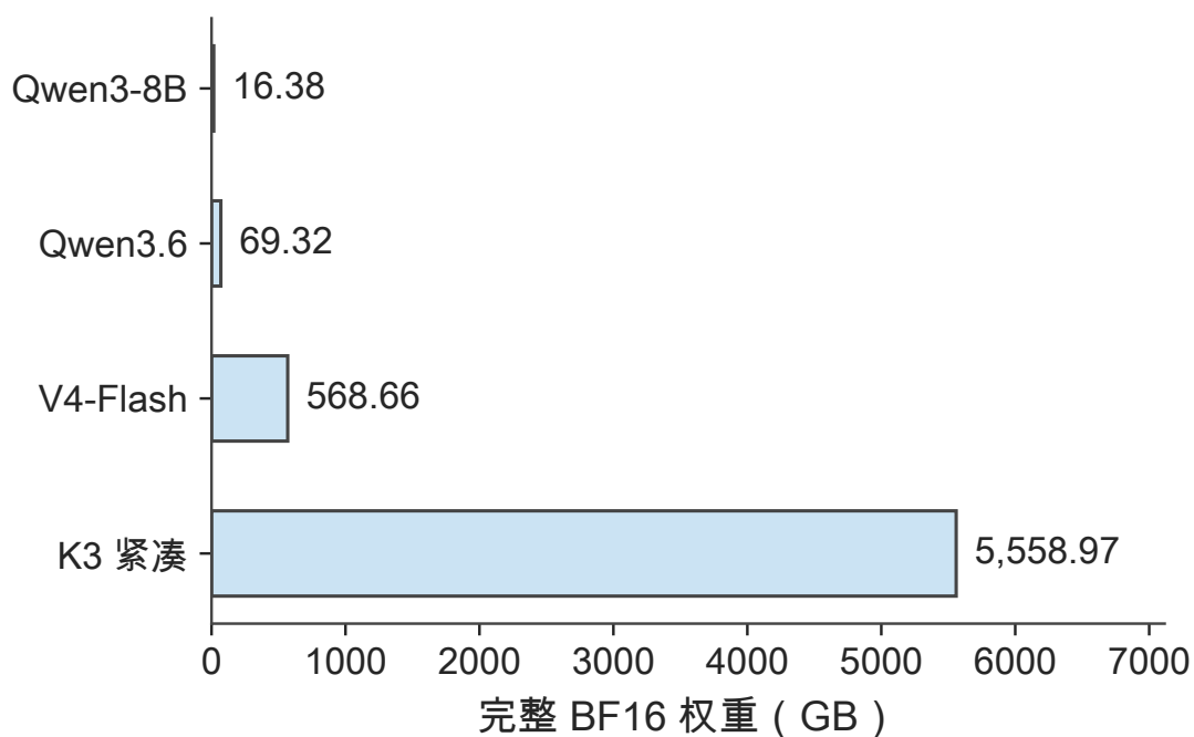
图 2-25 四模型完整权重统一用 BF16 表示时的容量，使用同一线性尺度。这里累计全部参数，包括每次仅选中部分的路由专家。
