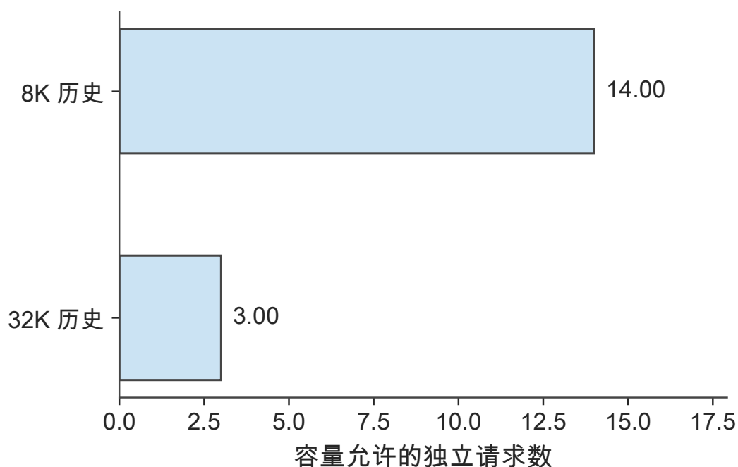
图 2-30 70B 的 4-bit 方案在同一张 80 GB 设备上，历史长度从 8K 增至 32K 时允许保留的独立请求数。每请求状态增加，使剩余空间容纳的请求数减少。
