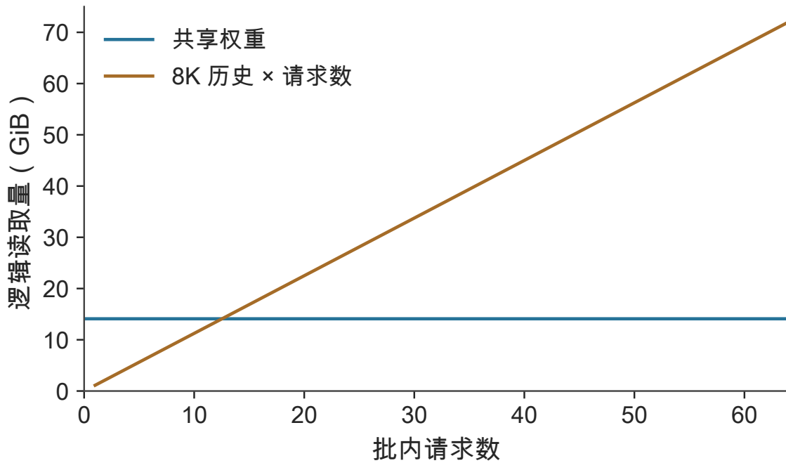
图 2-8 同一批次的主要投影权重可共享读取，各请求则各有一份历史。图中固定每请求 8K 历史，分别累计共享权重与独立 KV 的逻辑读取量。
