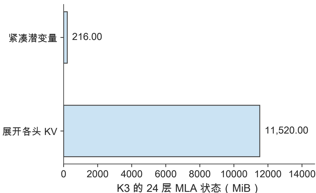
图 2-12 K3 的 24 层 MLA 在相同 8K 历史、BF16 下的两种保存量。紧凑路径保存上投影前的表示，展开路径保存各头的键和值。
