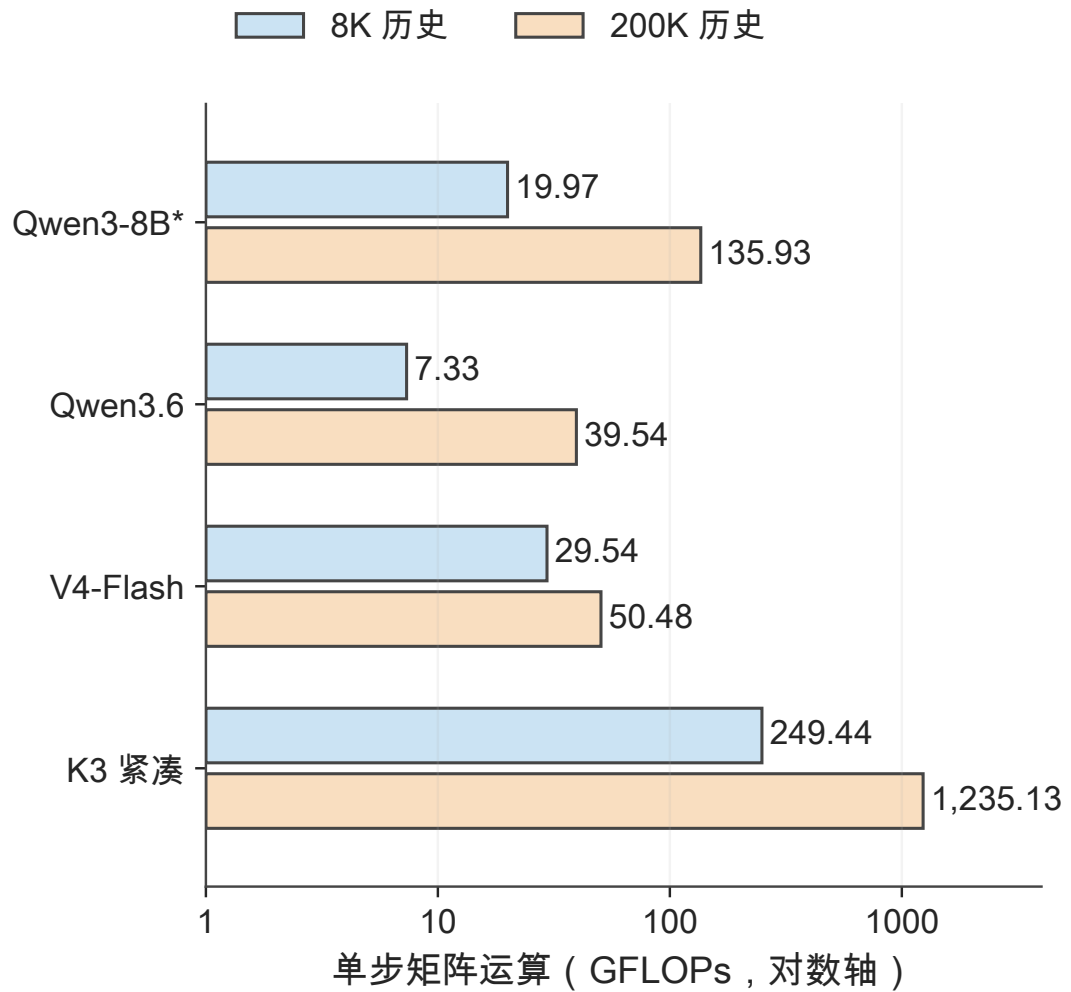
图 2-28 已有 8K / 200K 历史后再处理一个 token 的矩阵运算量。蓝、橙分别对应两种历史长度，横轴为对数刻度，柱端标出 GFLOPs。沿用表 2-C 的 decode 路径，K3 的 KDA 使用递推、MLA 使用紧凑表示。星号表示 Qwen3-8B 的 200K 条件超过本章固定配置的未缩放上下文上限，仅按原结构外推。
