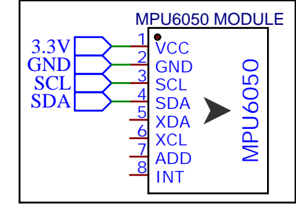
GIROSCOPIO/ACELEROMETRO
