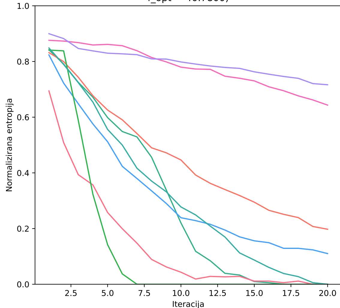
Normalizirana entropija skozi iteracije — F21_l1, dim 2 f_opt = 40.7800)
