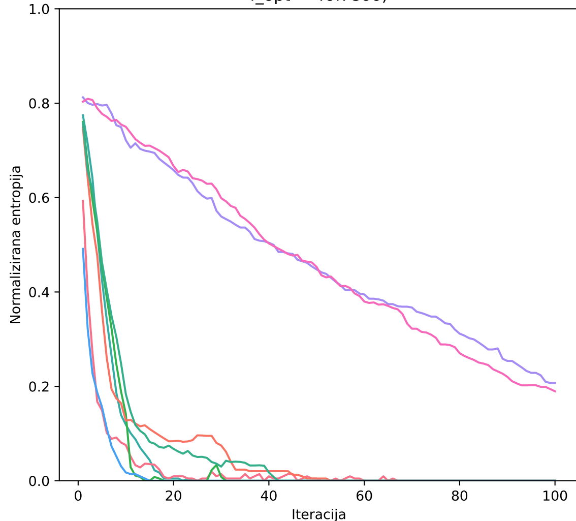
Normalizirana entropija skozi iteracije — F21_I1, dim 10 f_opt = 40.7800)
