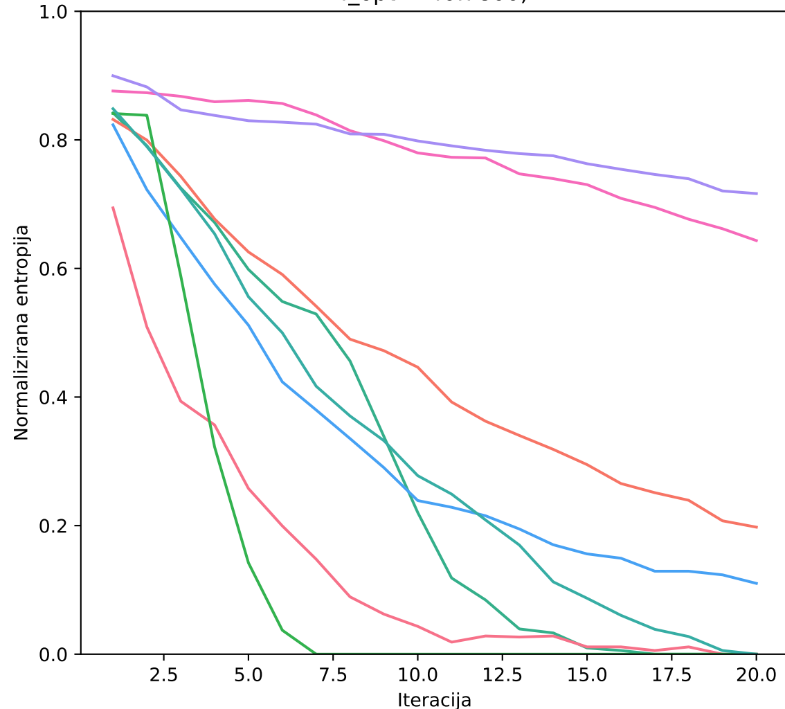
Normalizirana entropija skozi iteracije — F21_l1, dim 2 f_opt = 40.7800)
