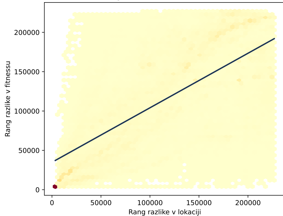
Dimenzija 2 ( \rho = 0.69 , n = 226800 )
