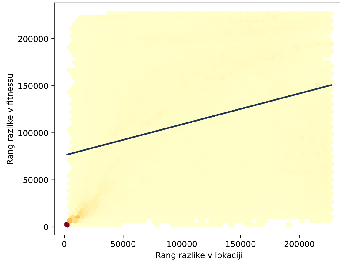
Dimenzija 5 ( \rho = 0.33 , n = 226800 )
