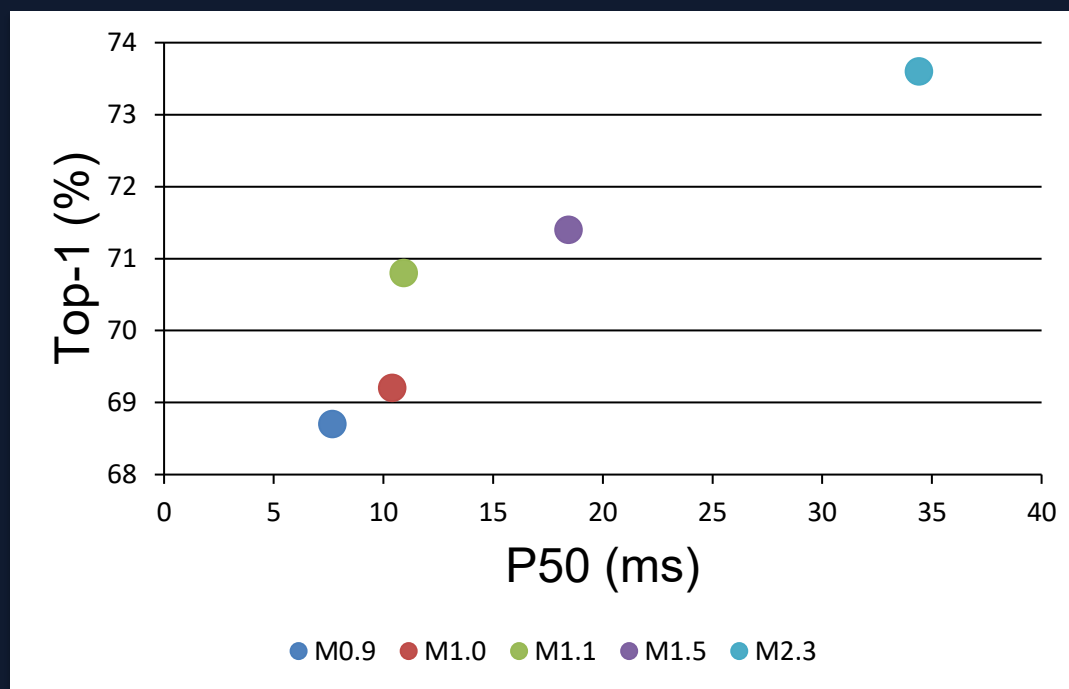
ImageNetV2 固定子集 (1000 张)：速度与准确率
